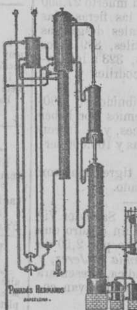
Aparato destilación continua á vapor. Producción del alcohol de 95 á 96°, ó sean 40° Cartier.
