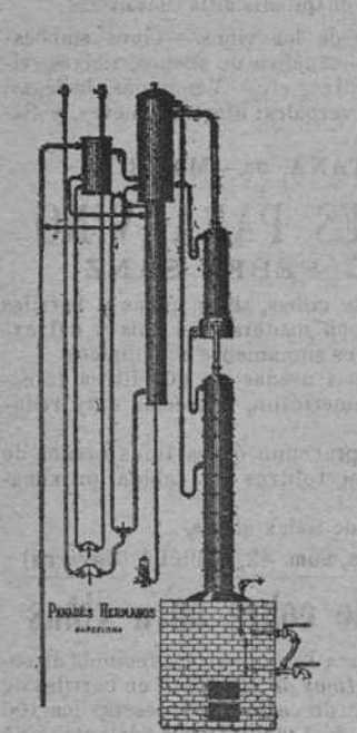
Aparato destilación continua á fuego directo. Producción del alcohol de 95 à 96°, ó sean 40° Cartier.
