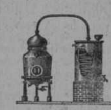
Alambique de vapor fijo ó basculante para Licores, Perfumes y Extractos
