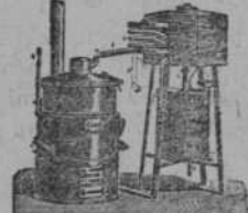
Alambique rectificador basculante, con calentamiento.—Da 80° Rapidez y economía
