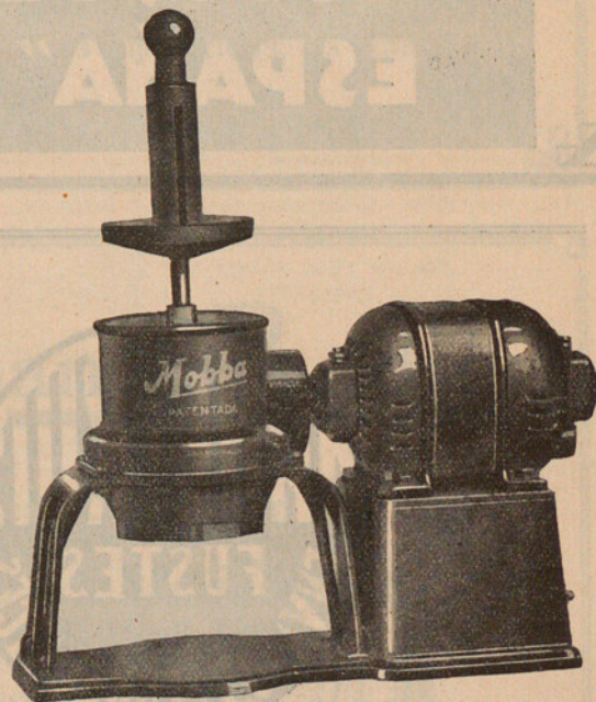
RATLLADORA DE FORMATGE
