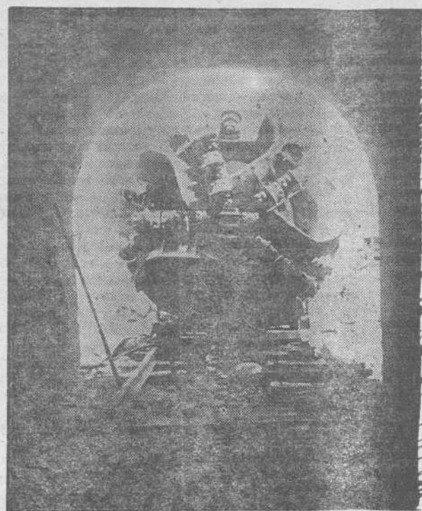
Cabeza cortadora del topo con sus tallantes. Una máquina prodigiosa para la obra del trasvase.
