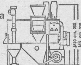
MOLINO MEZCLADOR M-5 Y-M-10 CON BASCULA Y SINFIN DE CORRECTORES
