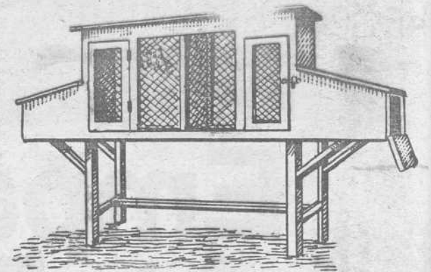
En la explotación familiar la jaula de conejos facilita el manejo de éstos, la parición y la limpieza de excrementos.
