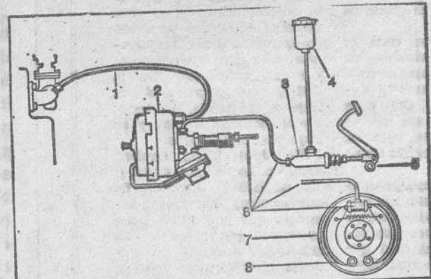
Esquema de un servofreno: 1, tubo de vacío del colector de admisión a la cámara del servo; 2, servofreno; 3, cilindro principal de la instalación hidráulica; 4, depósito de líquido de frenos; 5, pedal de freno; 6, conductos de la instalación hidráulica; 7, tambor de freno; 8, zapatas de freno.
