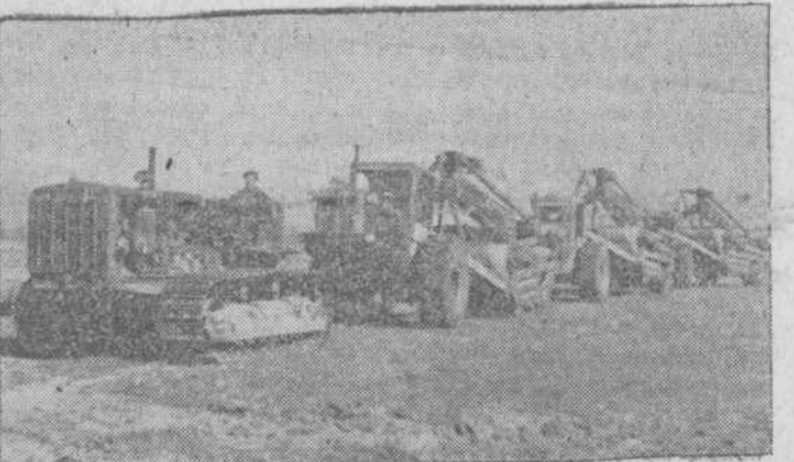
El tractor de arrastre y los tres grandes camiones-máquinas que ayer comenzaron, con extraordinaria rapidez y potencia, las obras de construcción de la primera pista de hormigón en el aeródromo de Matacán (Foto Guzmán Gombau.)
