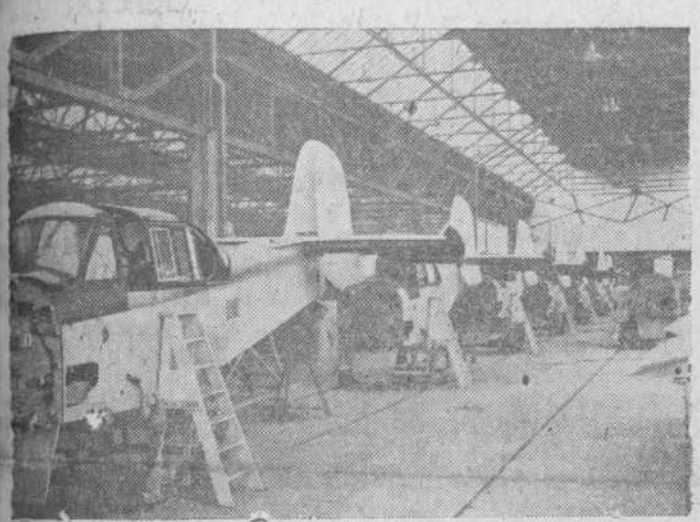
Aeroplanos Percival Prentice, que se están construyendo en Inglaterra, con destino a la Argentina, dispuestos en el taller de montaje para ser enviados a dicha nación
