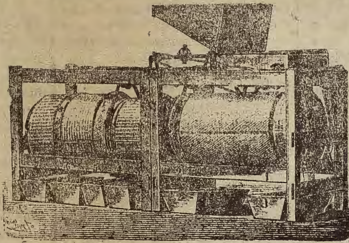
Seleccionadora Clert de doble divisor separador y volante
