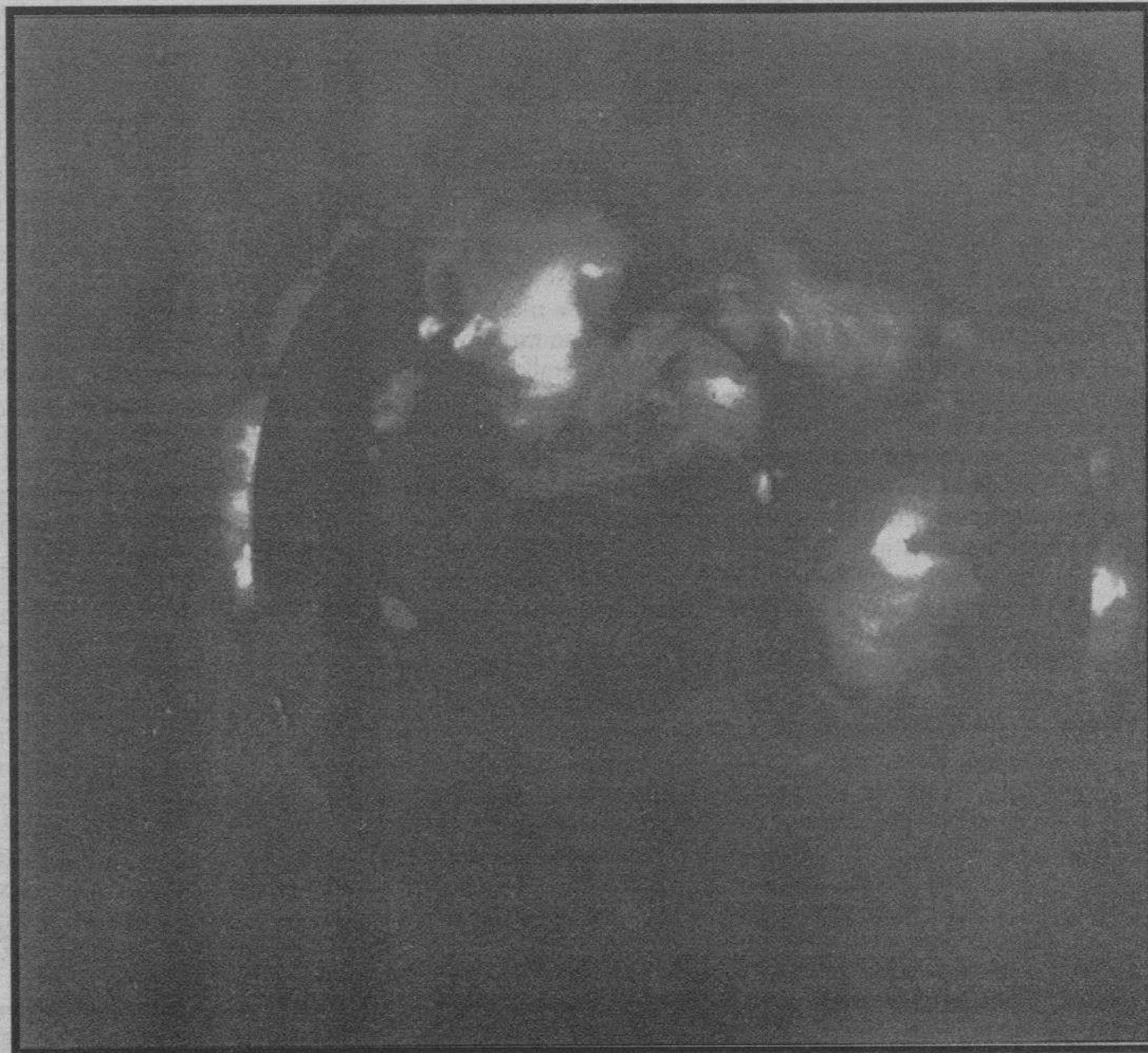
La imagen muestra las llamaradas emergentes de la superficie del Sol que ha detectado un telescopio de rayos X situado en el satélite japonés Yohkoh.
