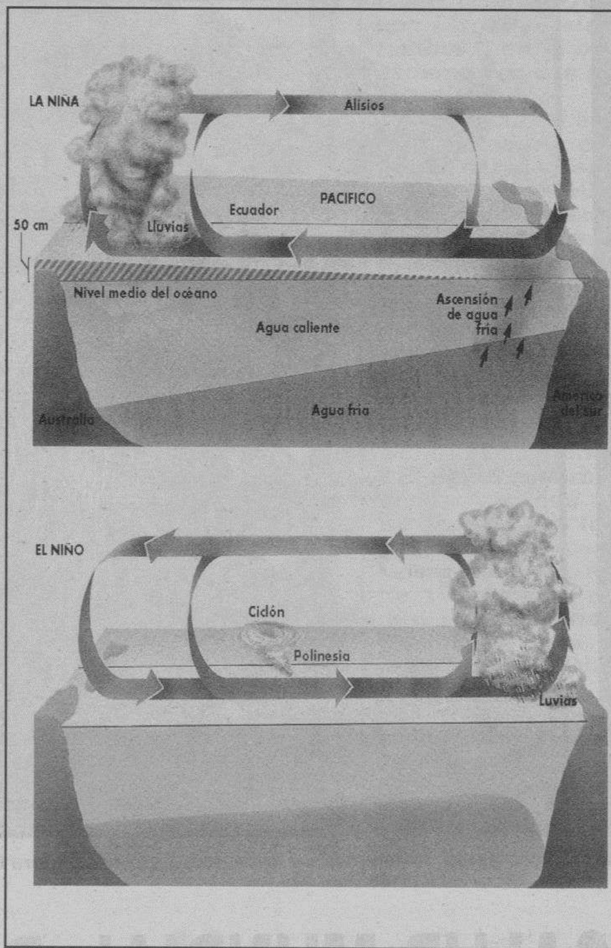
Mecanismo de "El Niño"
