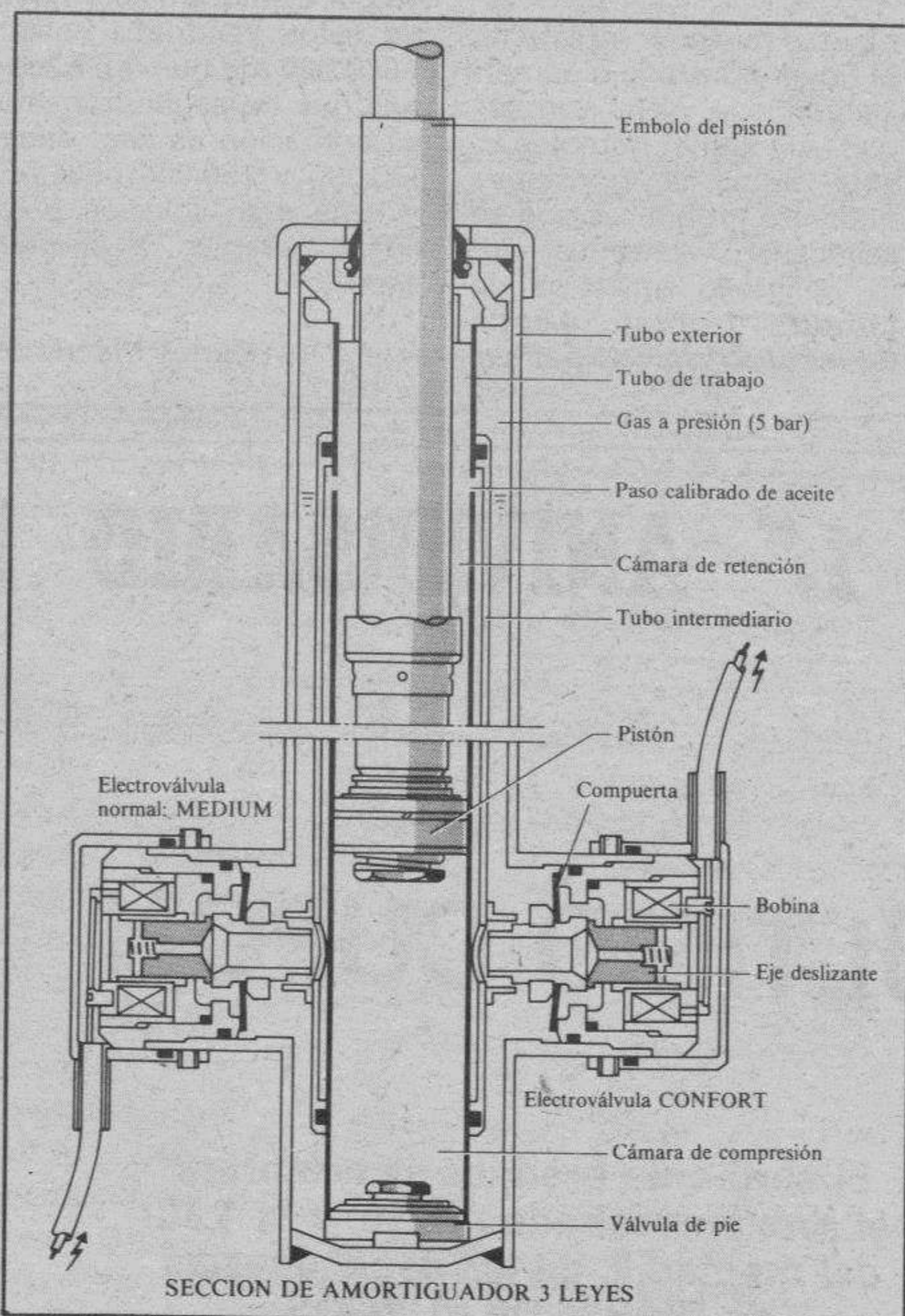
Esquema de la suspensión pilotada del Renault 25
