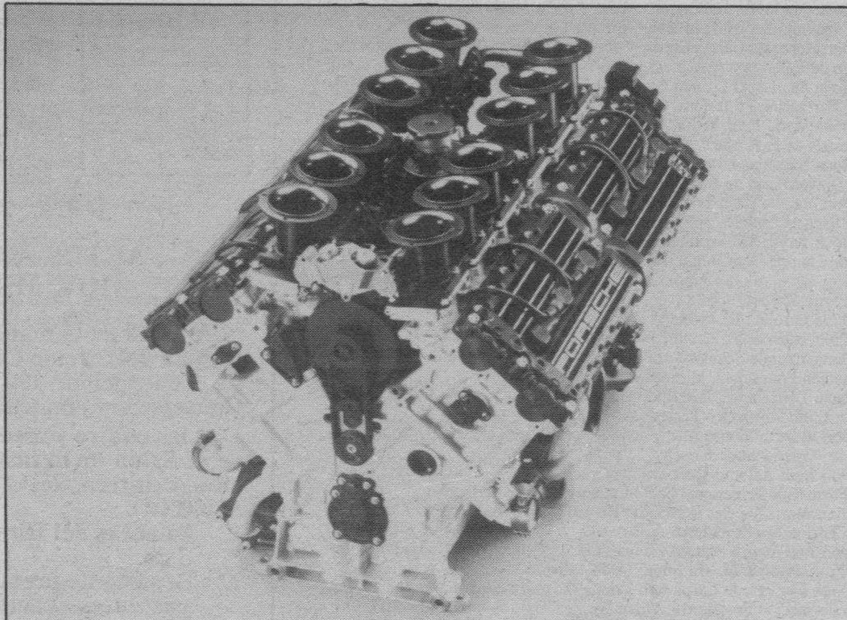
Motor Porsche para la Fórmula 1.- El nuevo motor que Porsche ha desarrollado para la Fórmula 1, tiene 3,5 litros y doce cilindros en V, con un ángulo de 80 grados. A partir de 1991, el equipo Footwork-Porsche competirá en el Campeonato del Mundo de Fórmula 1 con dos coches conducidos por Michele Alboreto y Alex Caffi
