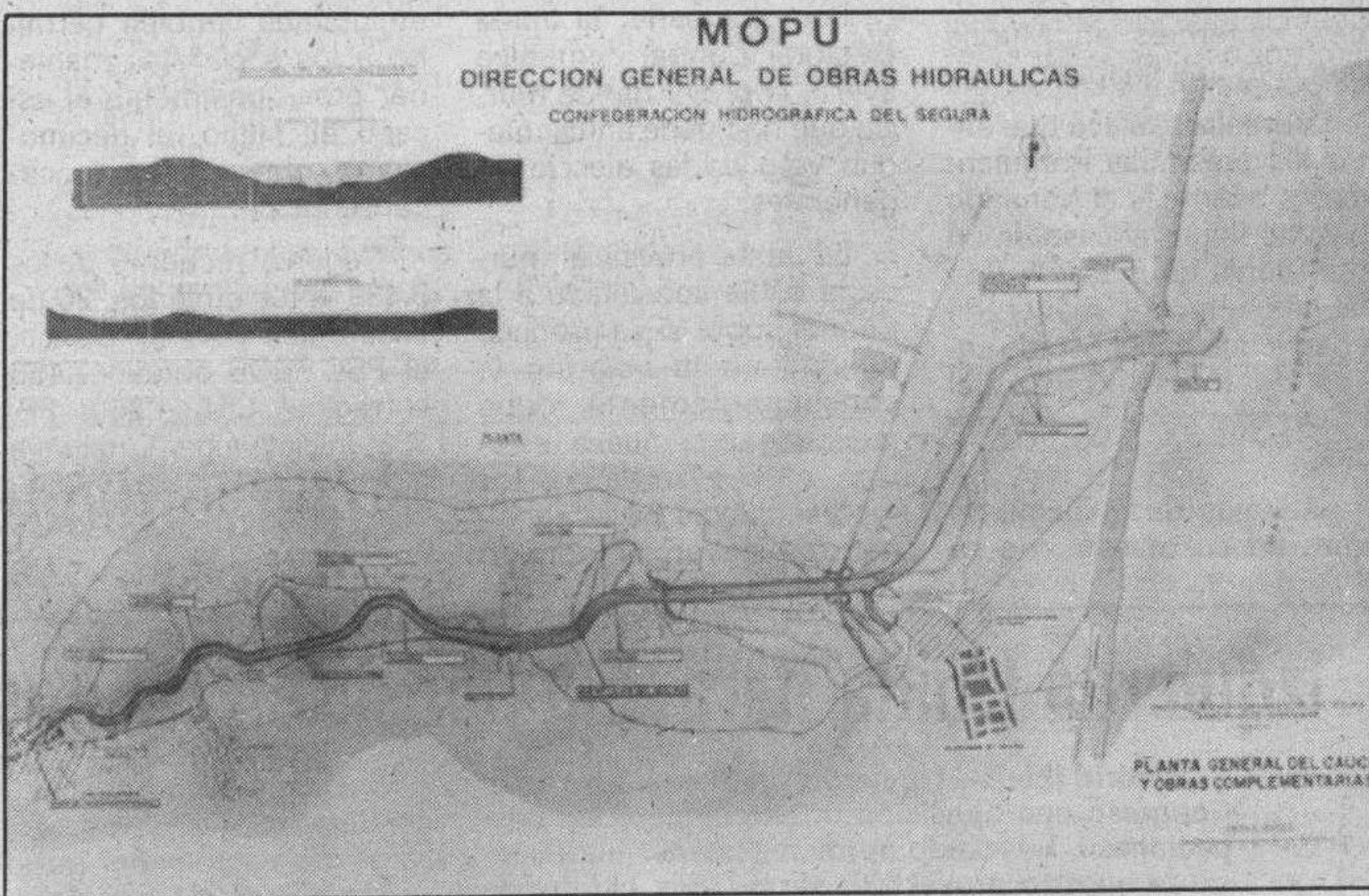
Plano del encauzamiento del Segura en la desembocadura. Efe
