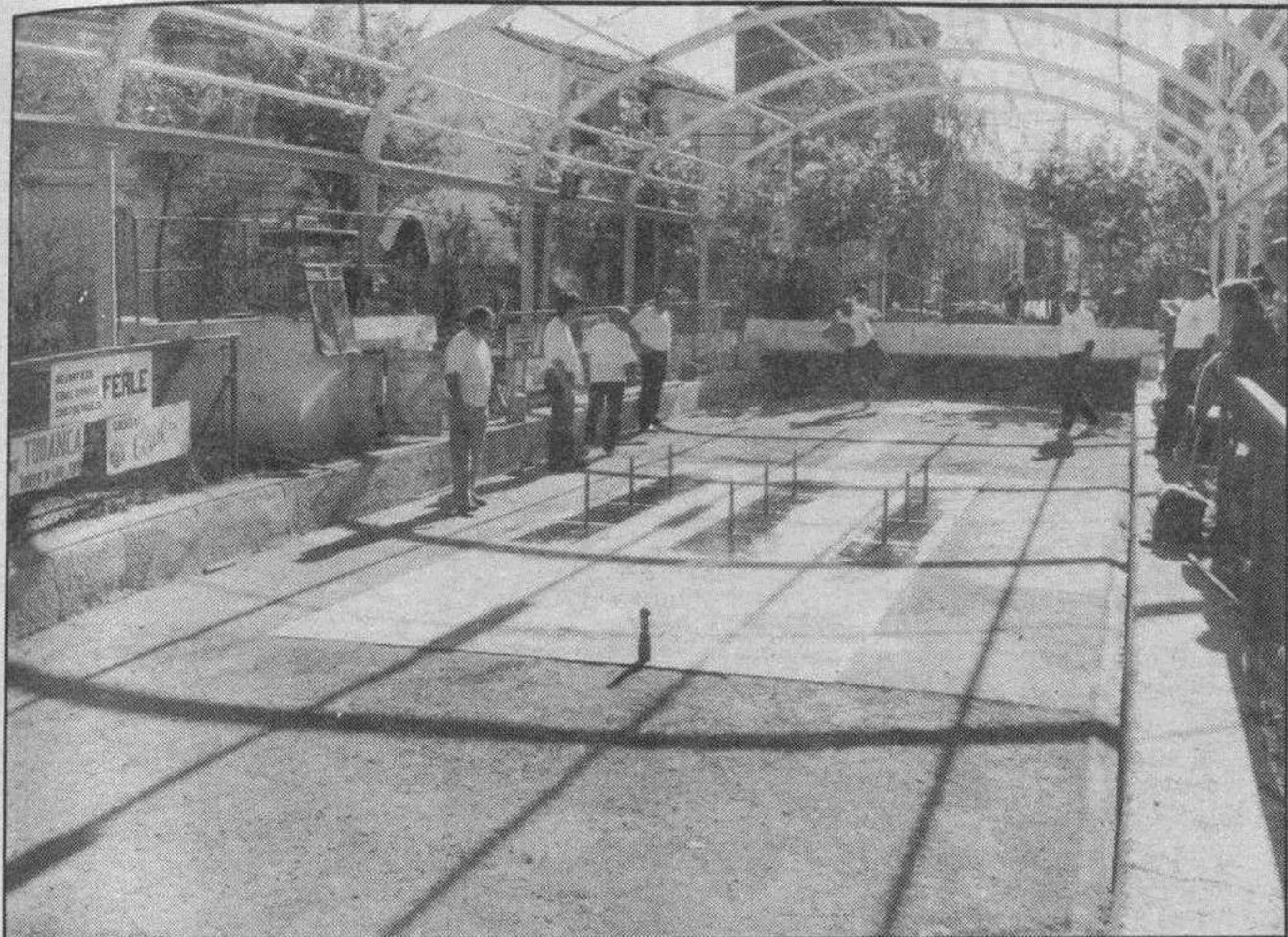
En la fotografía podemos apreciar la estructura de la cubierta de la Bolera Aquende, una estructura en arco. Se ha realizado la cubierta con poliéster blanco y azul, con ello no se eliminará la luz y sí el calor en verano y la lluvia o la nieve en invierno. Los trabajos han sido realizados en un plazo de mes y medio
