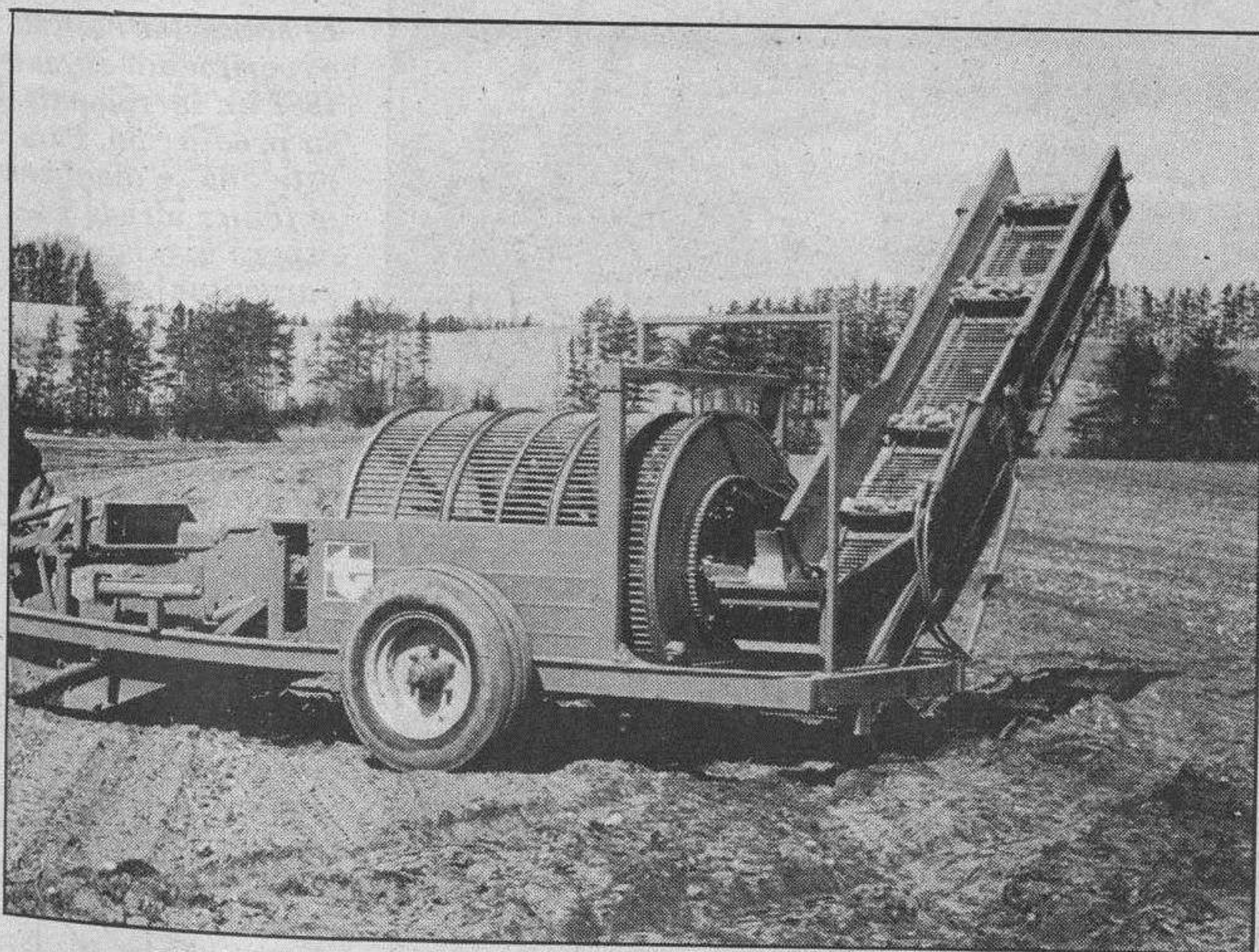
COSECHADORA INTEGRAL DE PATATAS
