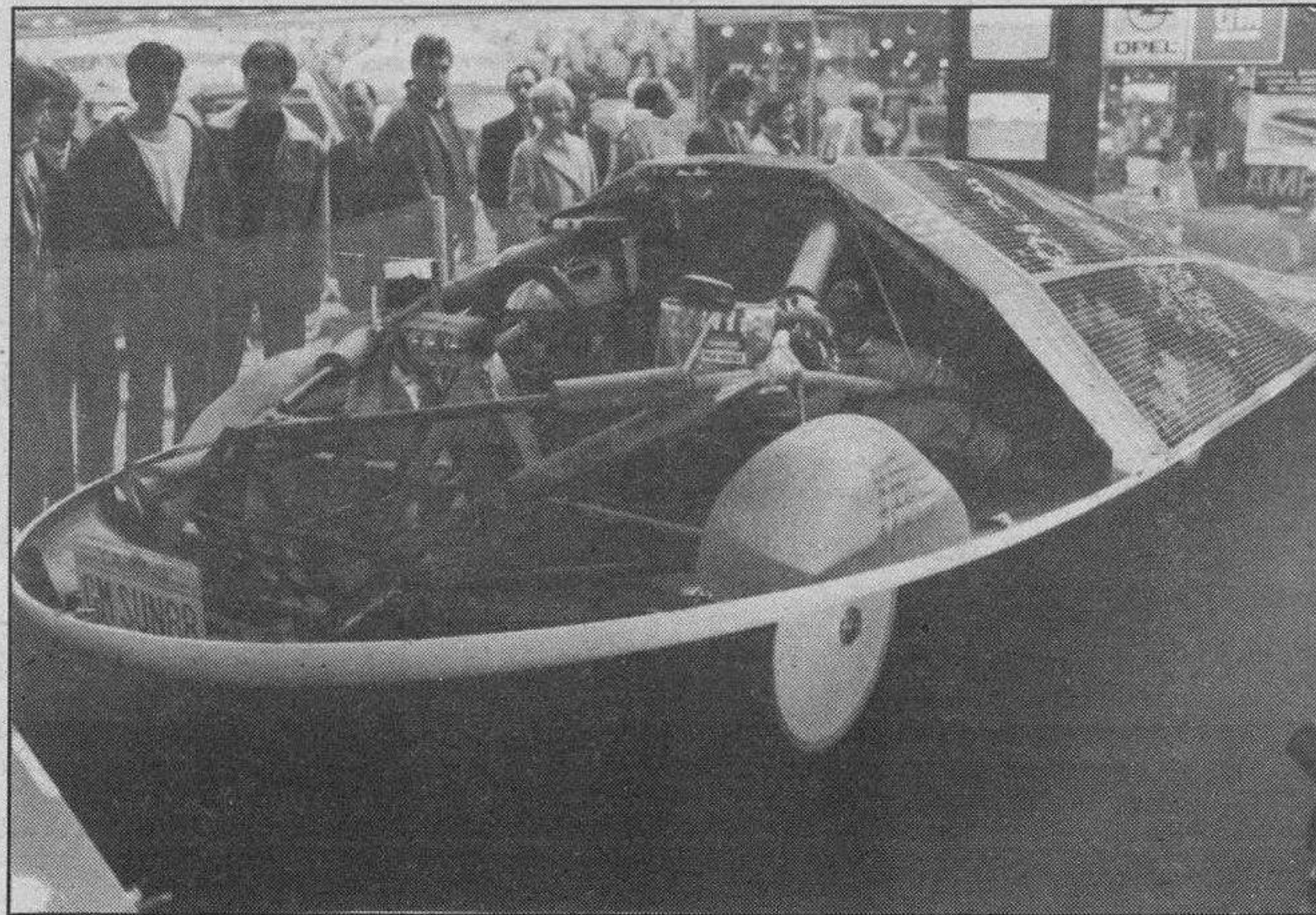
Este coche mide seis metros de largo, dos de ancho y uno de altura y su peso es de 260 kilos.
