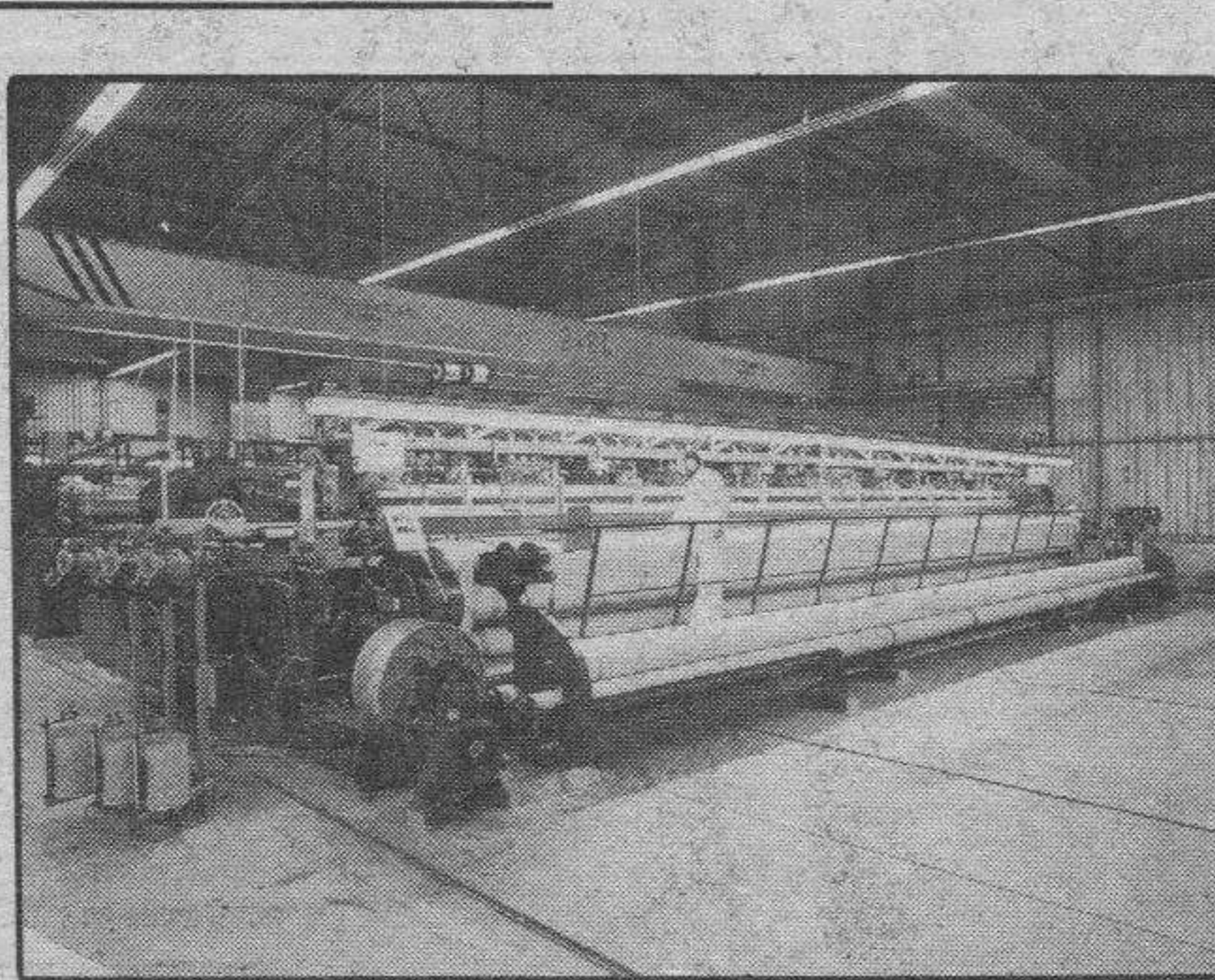
Proceso de fabricación de la gama de productos, telares y de termofijado en la calandra.
