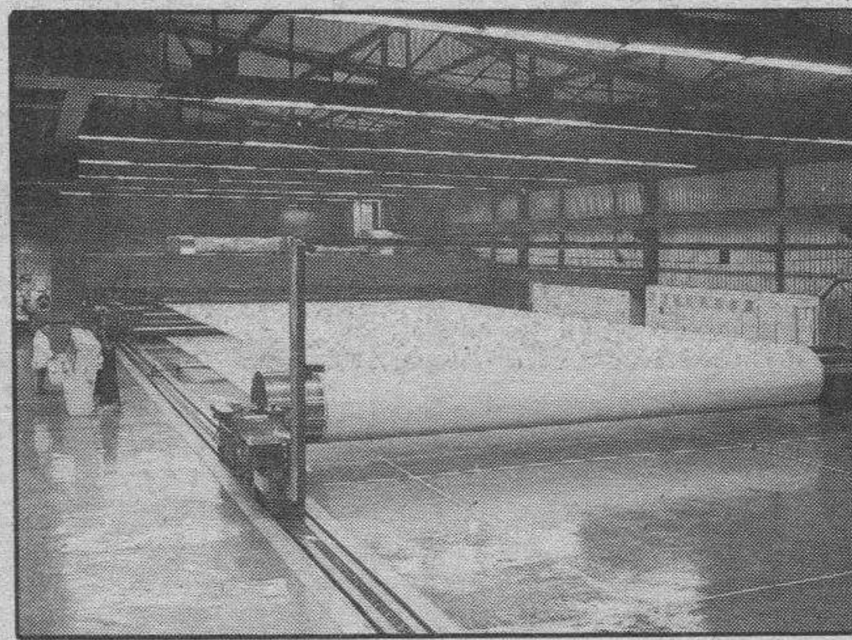
Proceso de fabricación de la gama de productos, telares y de termofijado en la calandra.
