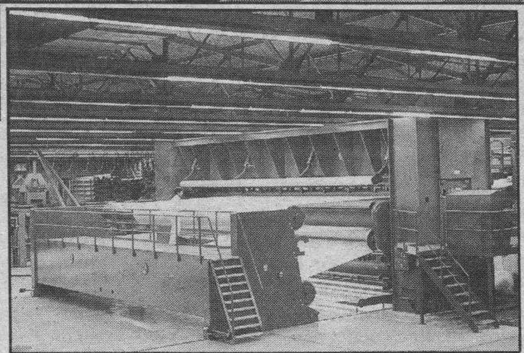
Fase de agujado de napa para fieltros.
