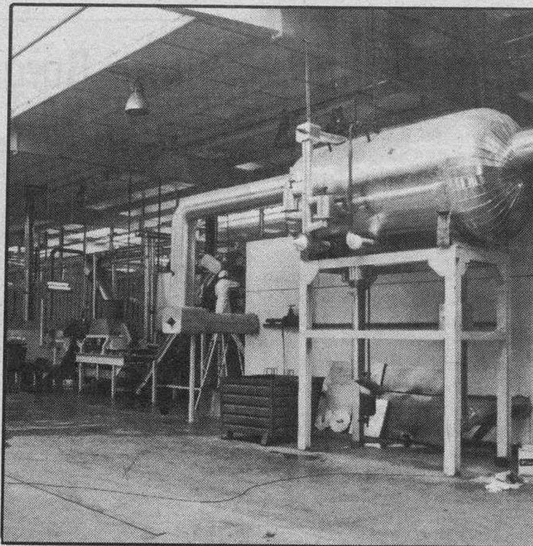
Línea de fabricación de la patata frita congelada
