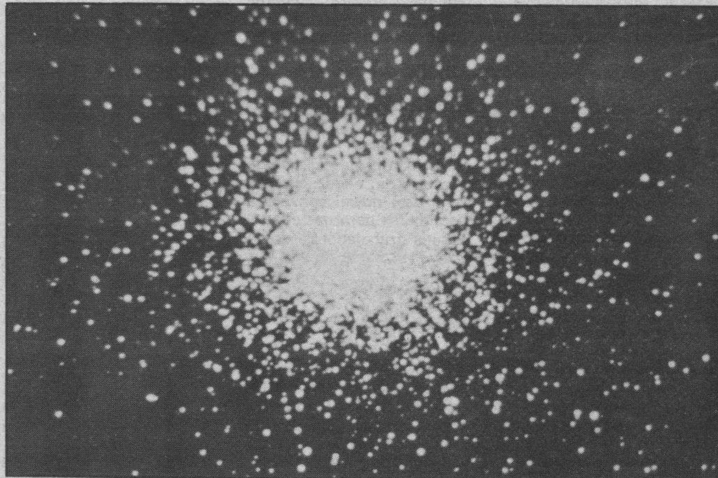
Típico ejemplo de cúmulo globular. Se trata de M13, en Hércules. Dista de nosotros 25.000 años-luz, y su diámetro es 170 años-luz. Contiene más de 100.000 estrellas
