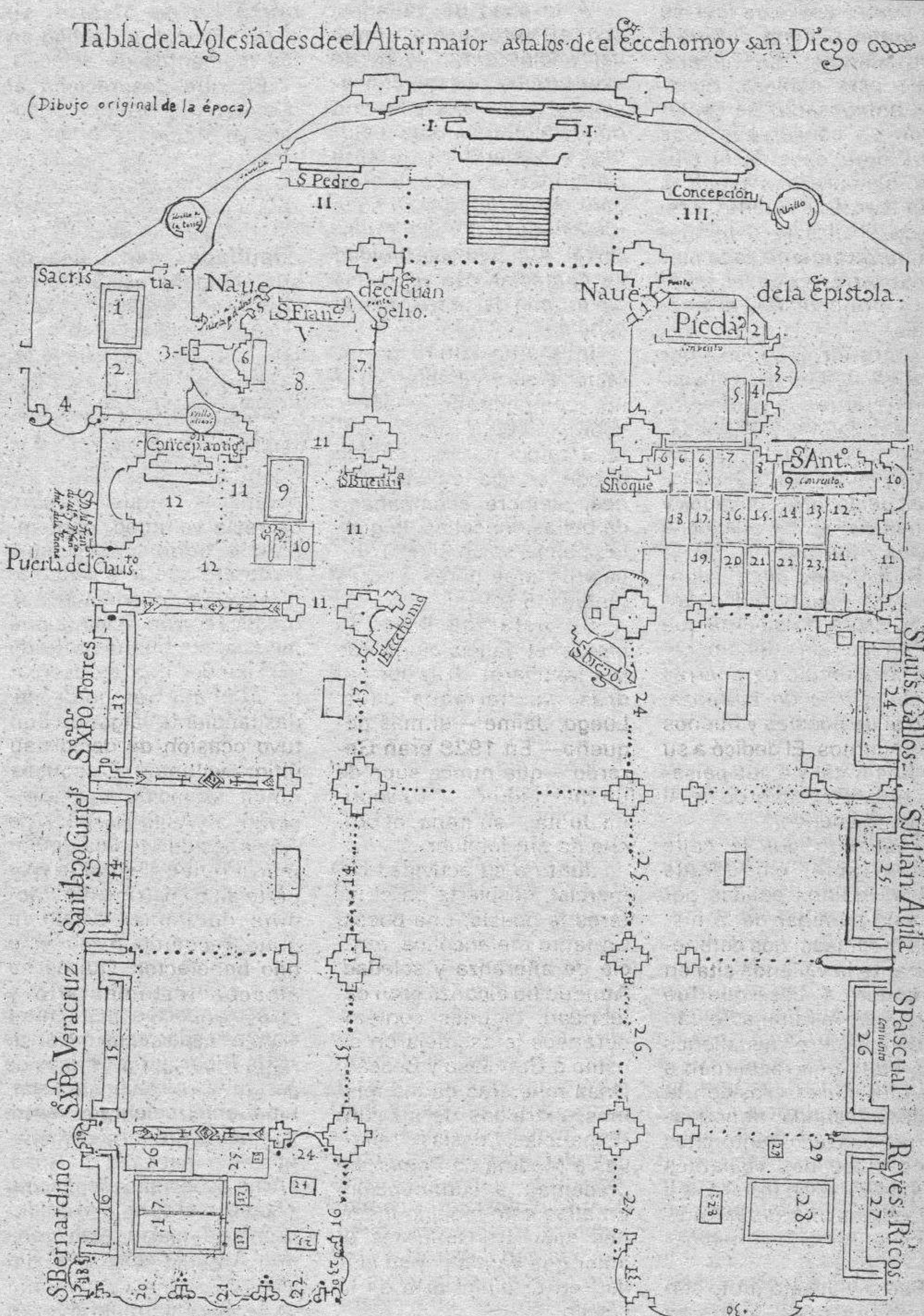
Planta del templo de S. Francisco en Burgos: capillas y dependencias en el siglo XVI
