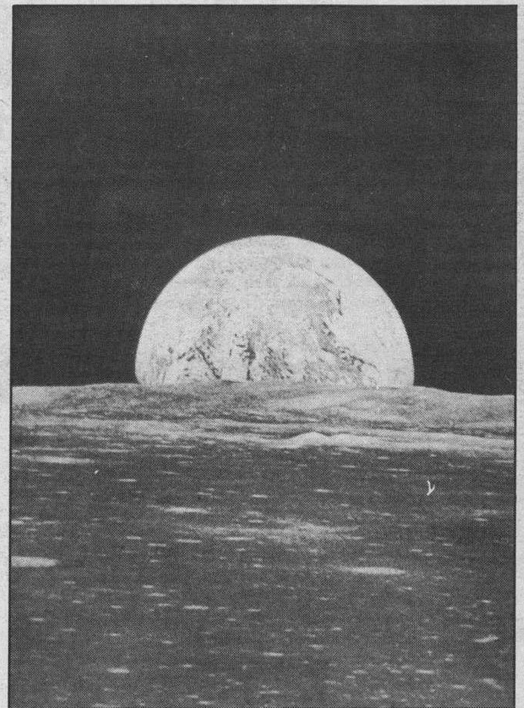
Fotografía de la Tierra desde la superficie lunar, obtenida en la última misión «Apolo», en 1972.
