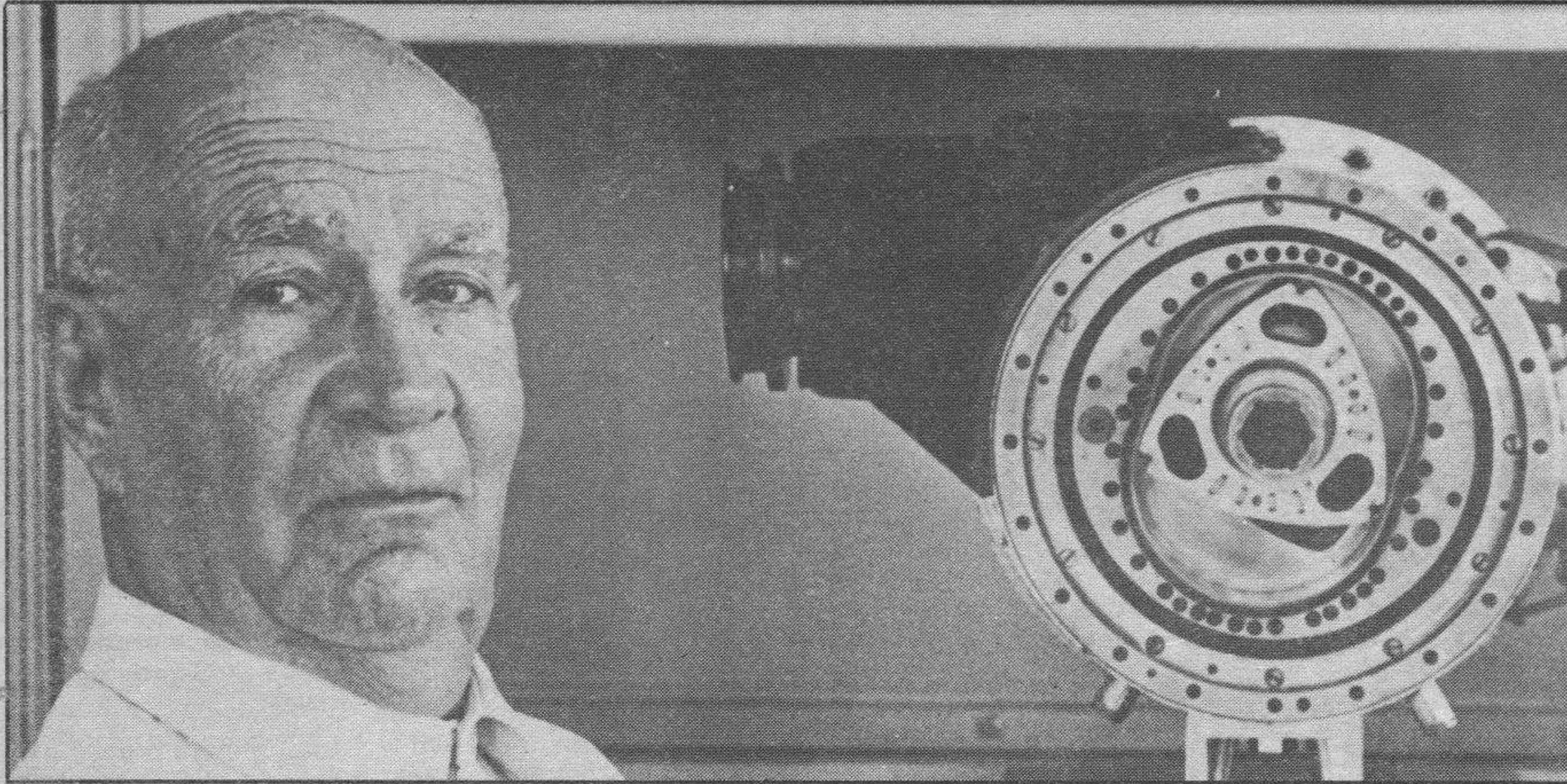
Inventor cumplió 85 años. — Félix Wankel, inventor del motor de pistón rotativo, celebró en Lindau, a orillas del Lago de Costanza (República Federal de Alemania), su 85 cumpleaños. A la derecha, un modelo en corte del motor que lleva su nombre. Wankel ha instalado en Lindau un Museo de motores digno de verse; es un genio infatigable que siempre logra desarrollar con éxito nuevas ideas.
