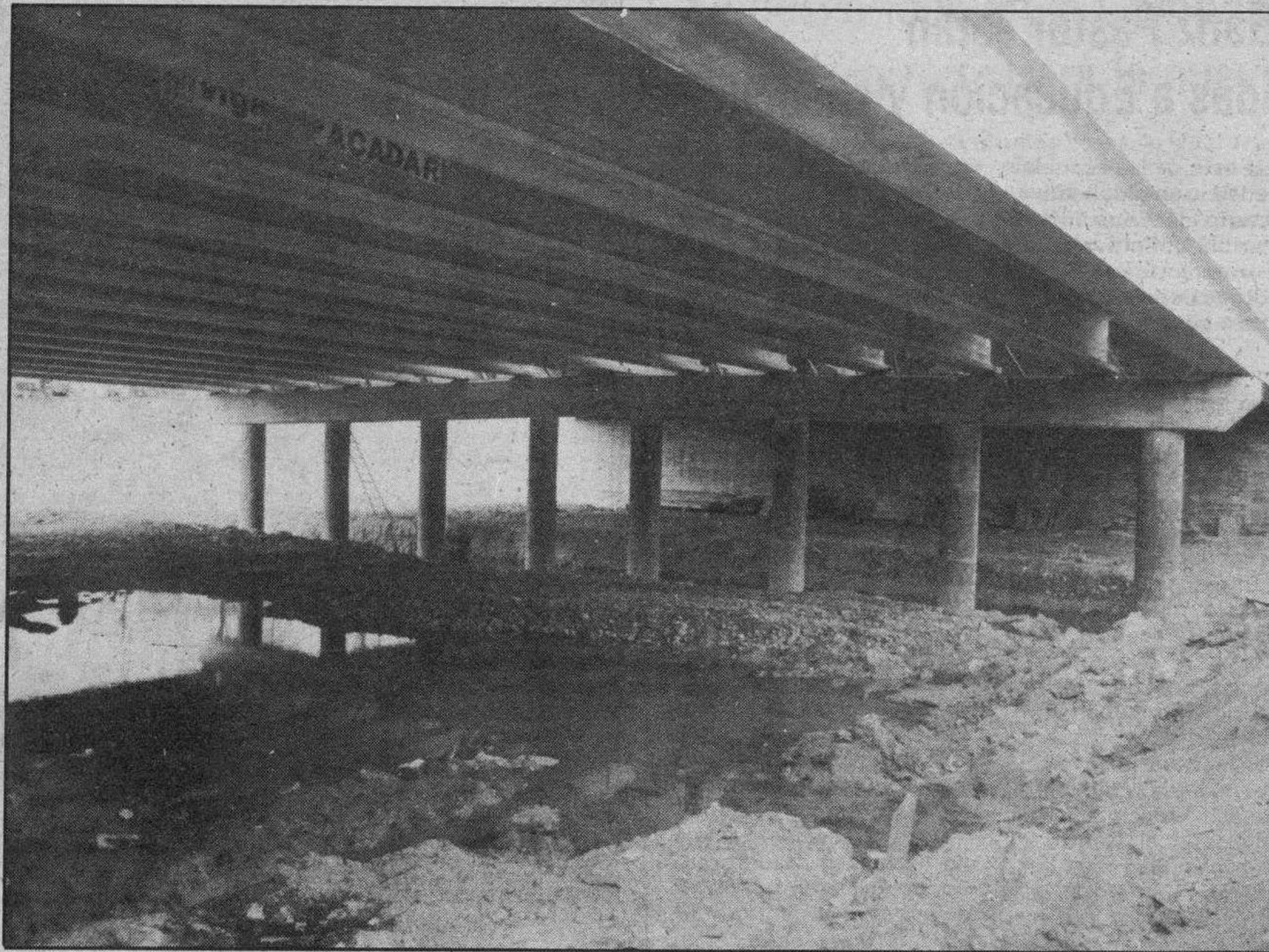
Estructura inferior del puente en el que se está trabajando.
