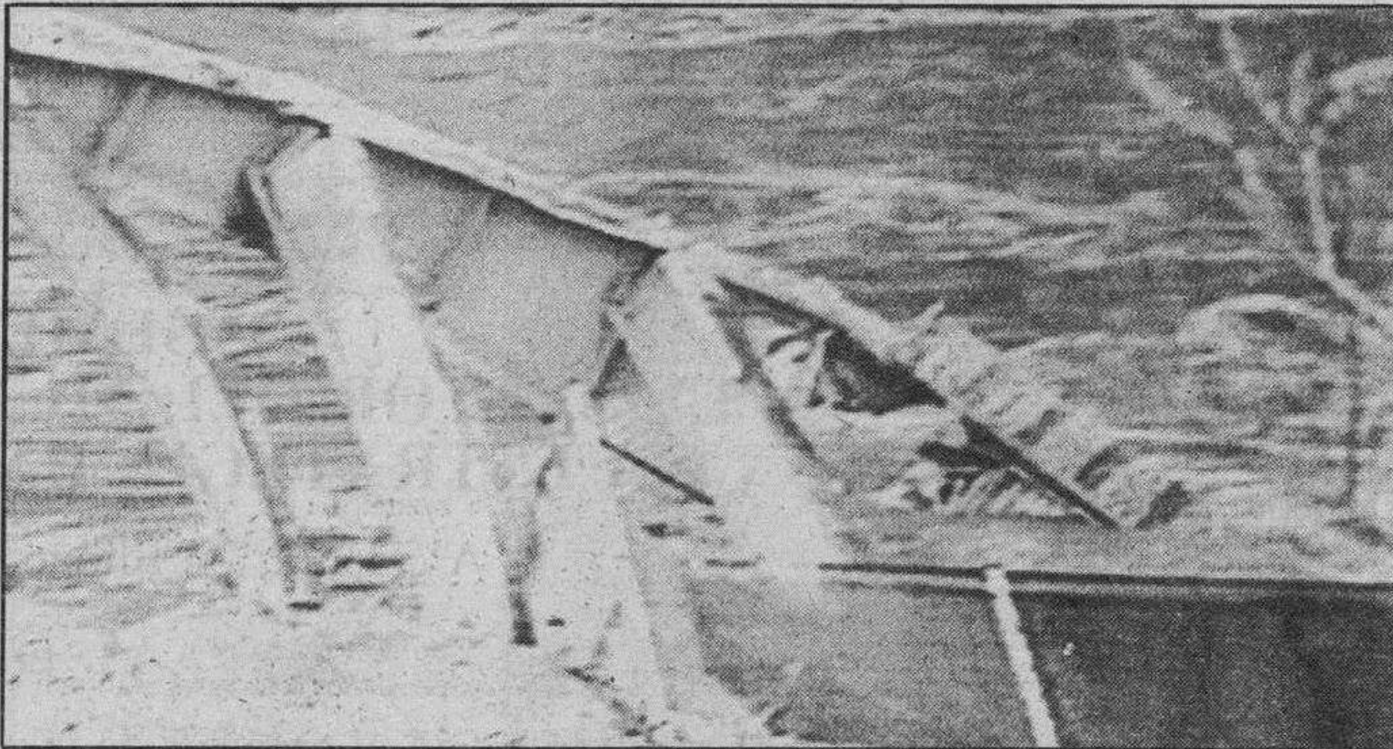
Estado en que quedó el puente, tras ser arrastrado por las aguas del río Schoharie Creek.
