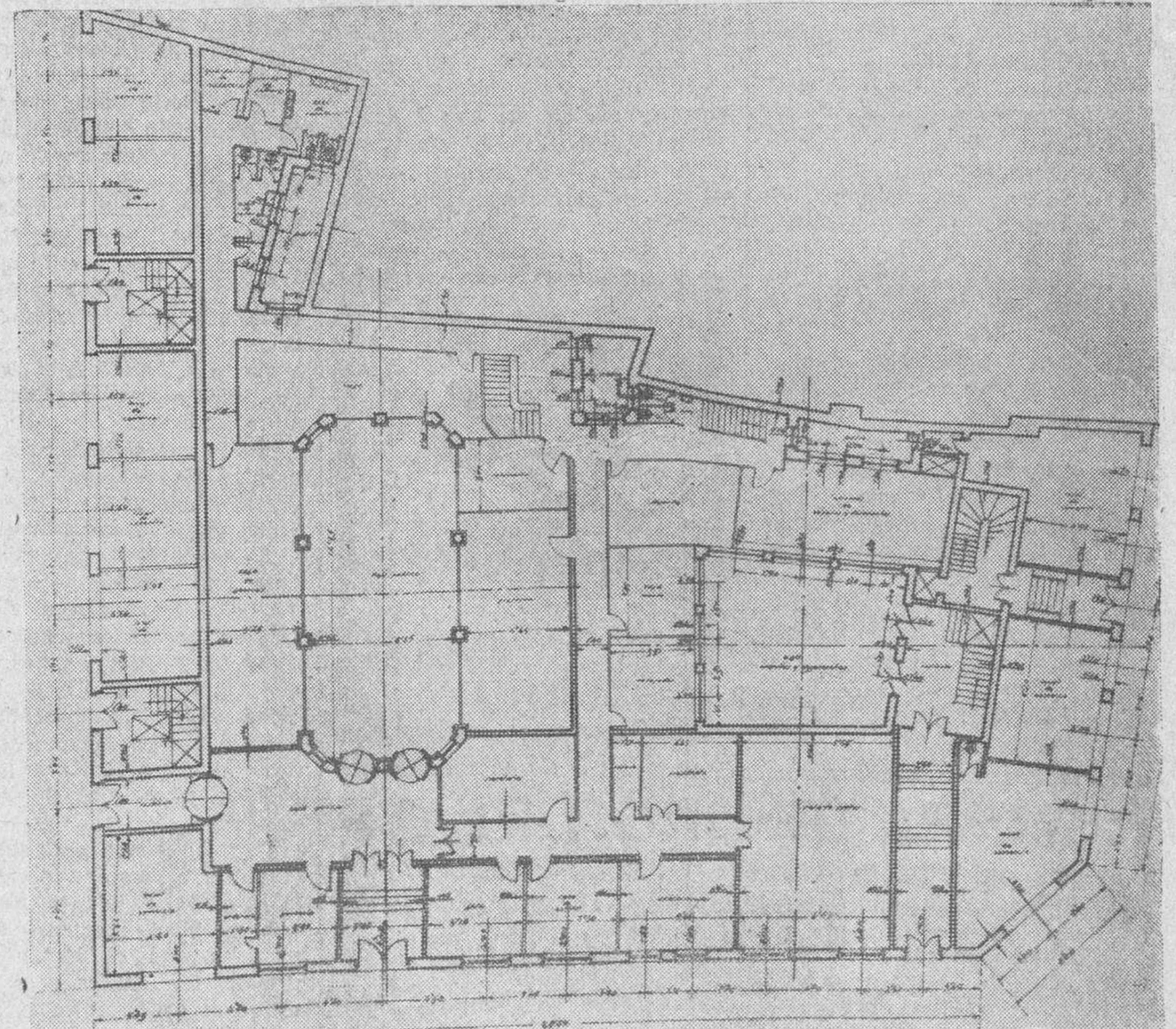
Planta baja del edificio, destinado a oficinas de la Caja de Ahorros y Monte de Piedad, con fachada a la calle de Espoz y Mina y al Pasaje
