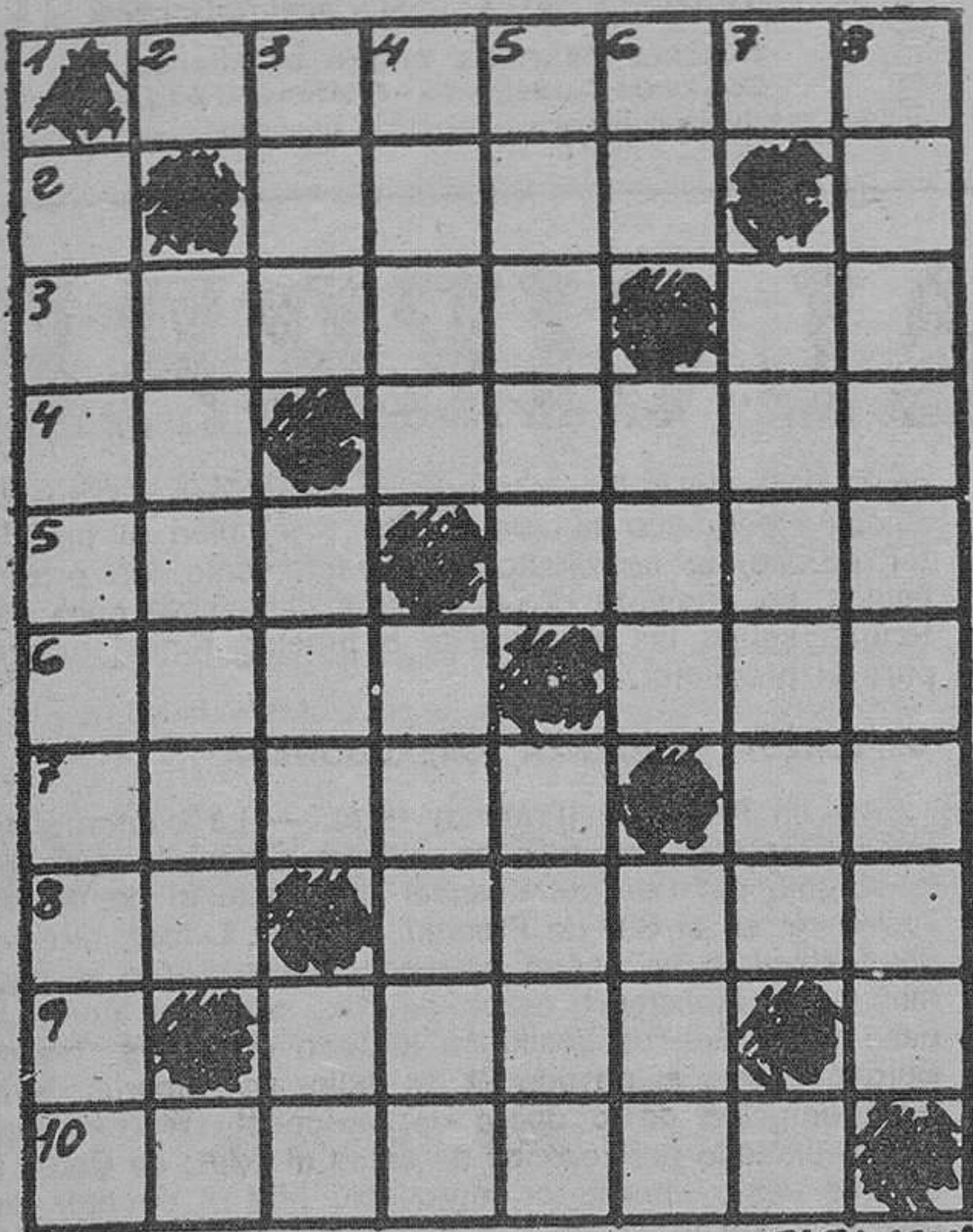
FIEL (FN)
