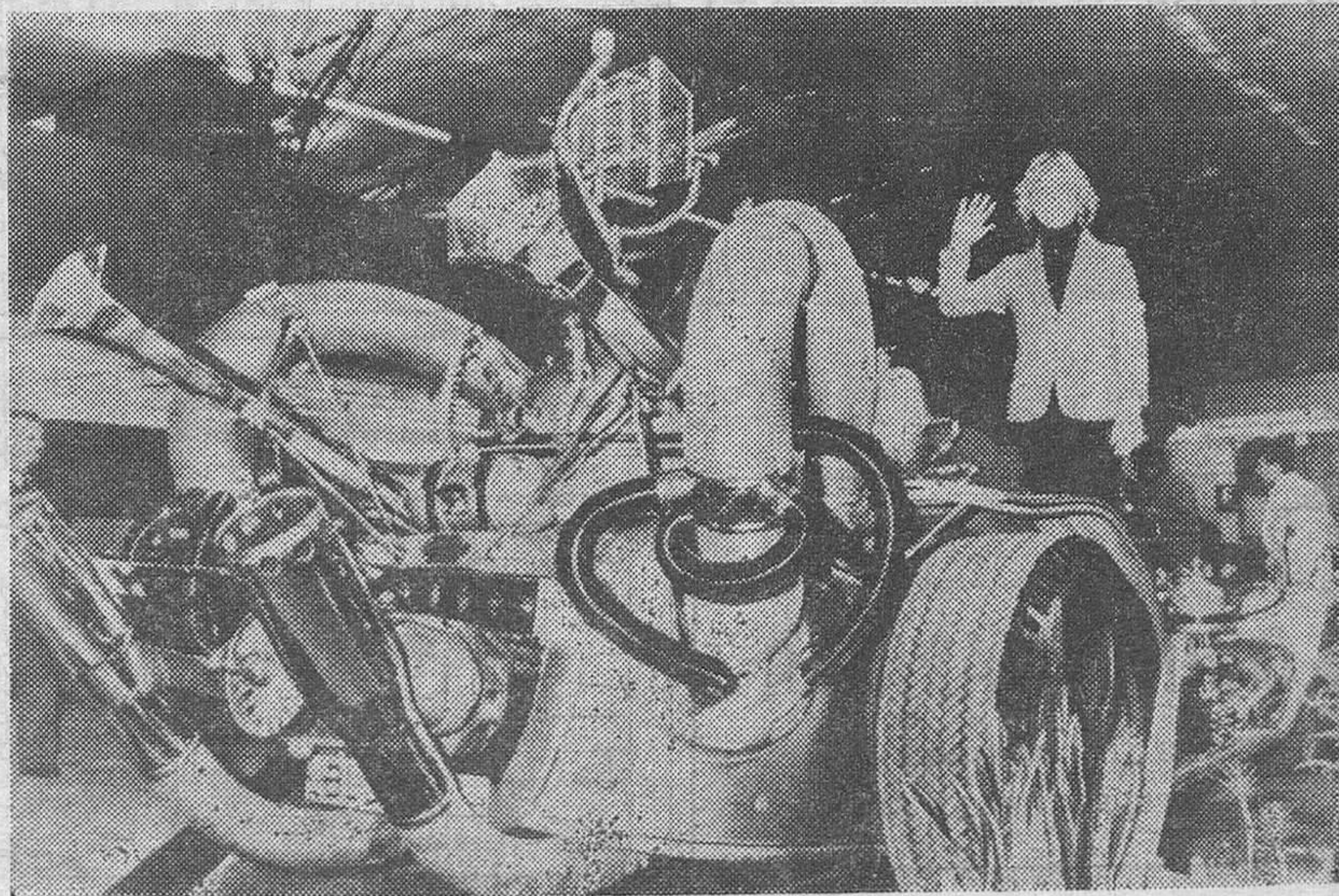
Ginebra (Suiza).— Este automóvil, llamado «El Tempo Gigante», que tiene 6,7 metros de largo por 2,1 de ancho y que es movido por dos motores, uno turbo. Ha sido construido en Noruega por el productor de cine Ivo Caprini. El coche se exhibe en la exposición de automóviles de Ginebra. — (Telefoto EFE-UPI)
