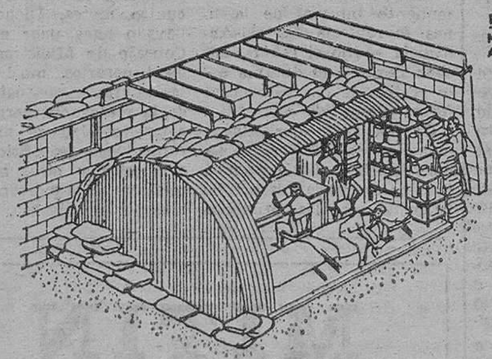
FIGURA 1. MOD. PLANCHAS DE ACERO CURVADOS
