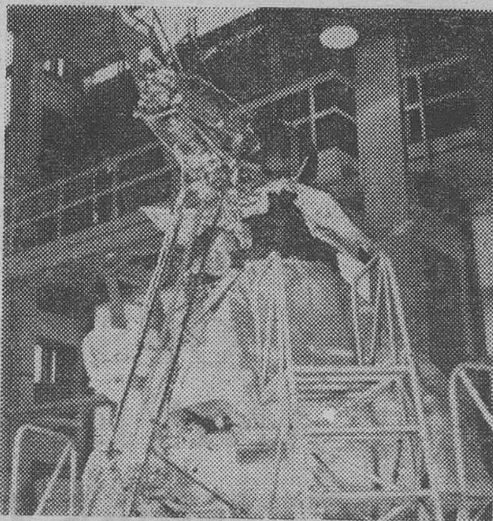
Moscú. — La foto muestra el bloque ensamblado de la estación automática "Luna-24". En primer término, el dispositivo de recogida de sedimentos de la superficie de la Luna
