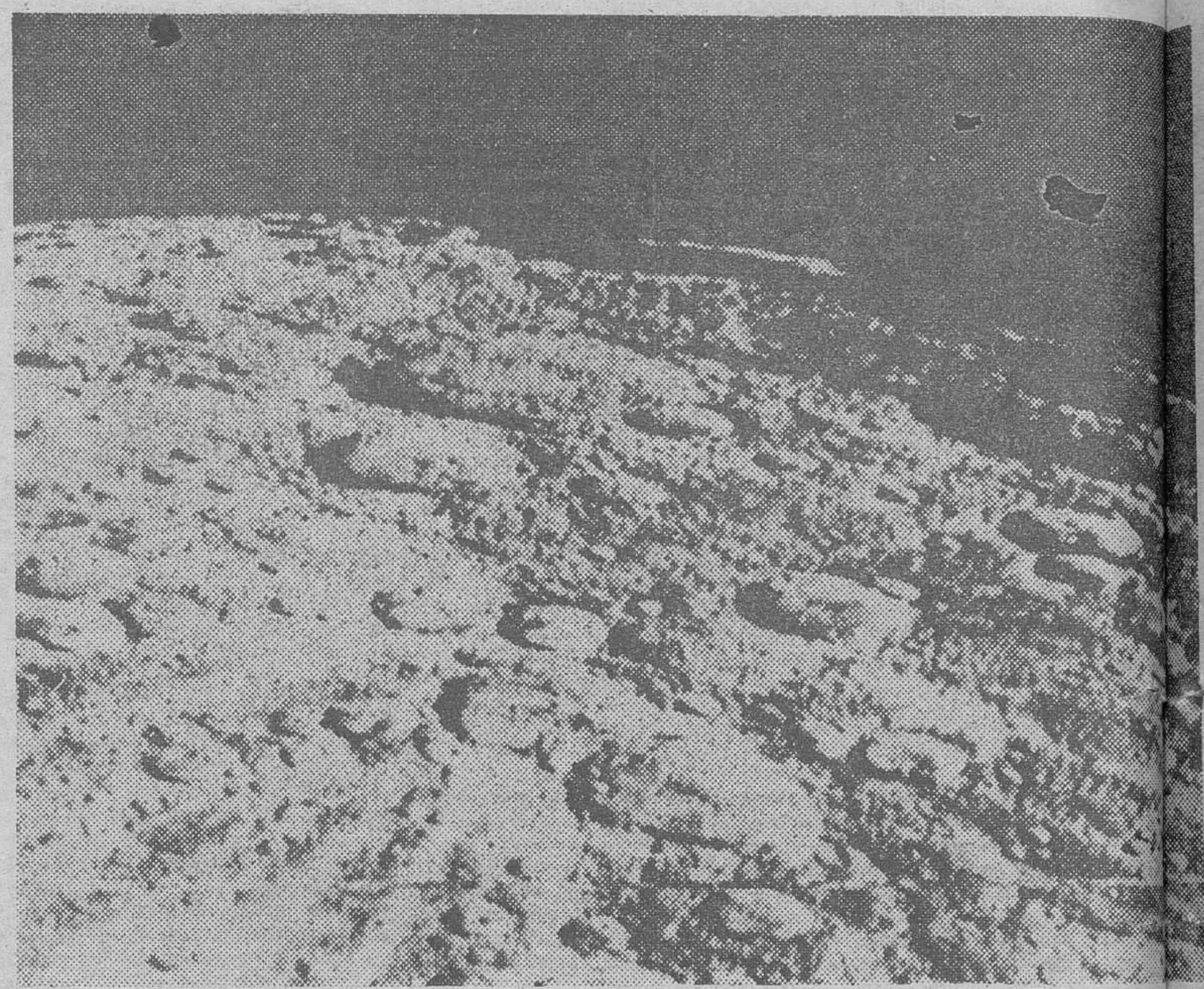
Aspecto "lunar" del Polo Sur de Mercurio, según detallada fotografía tomada desde 85.000 kilómetros del planeta, por la sonda norteamericana «Mariner 10». — (Foto EFE)
