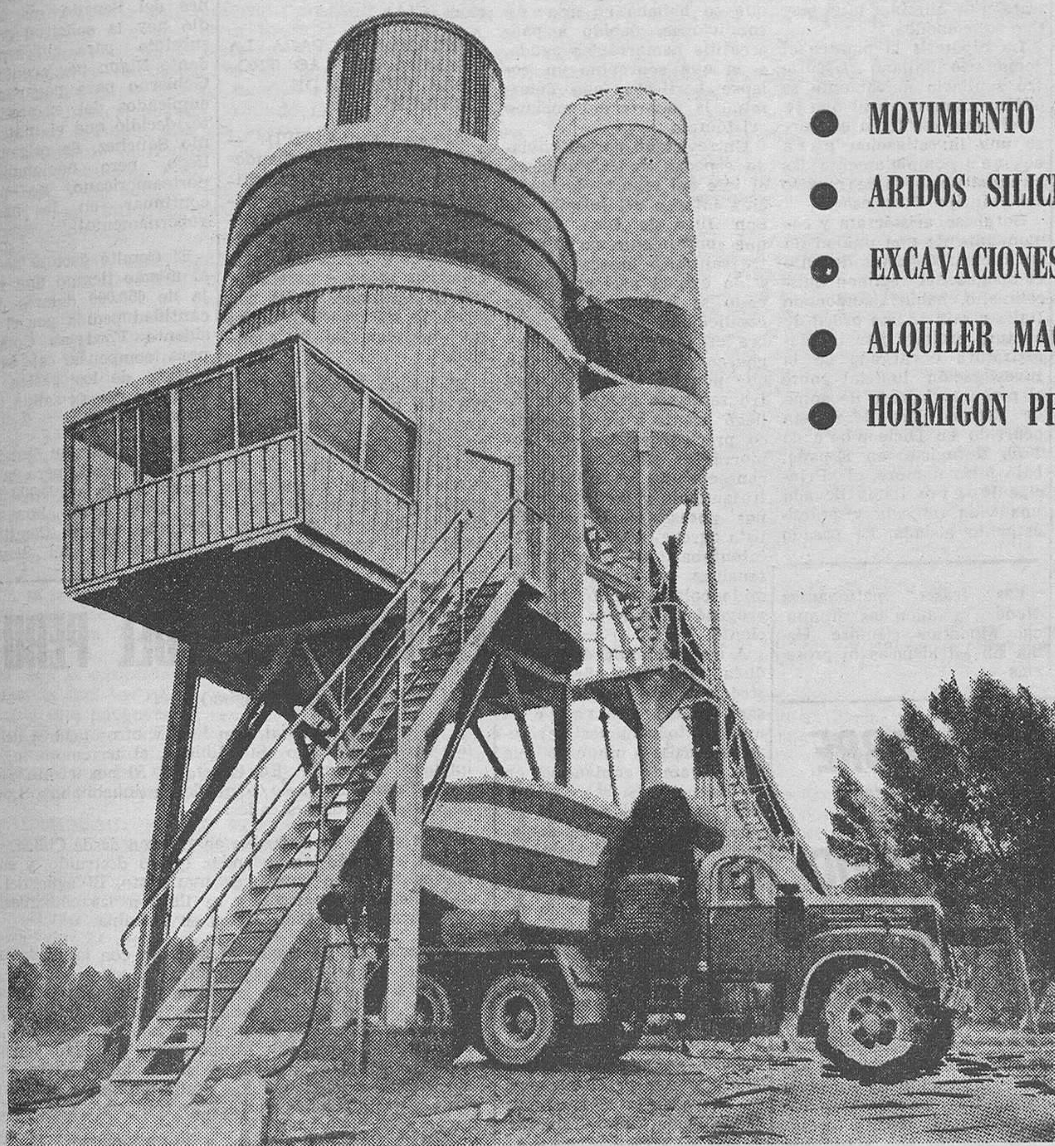
Central automática de hormigón para 135 m 3 hora
