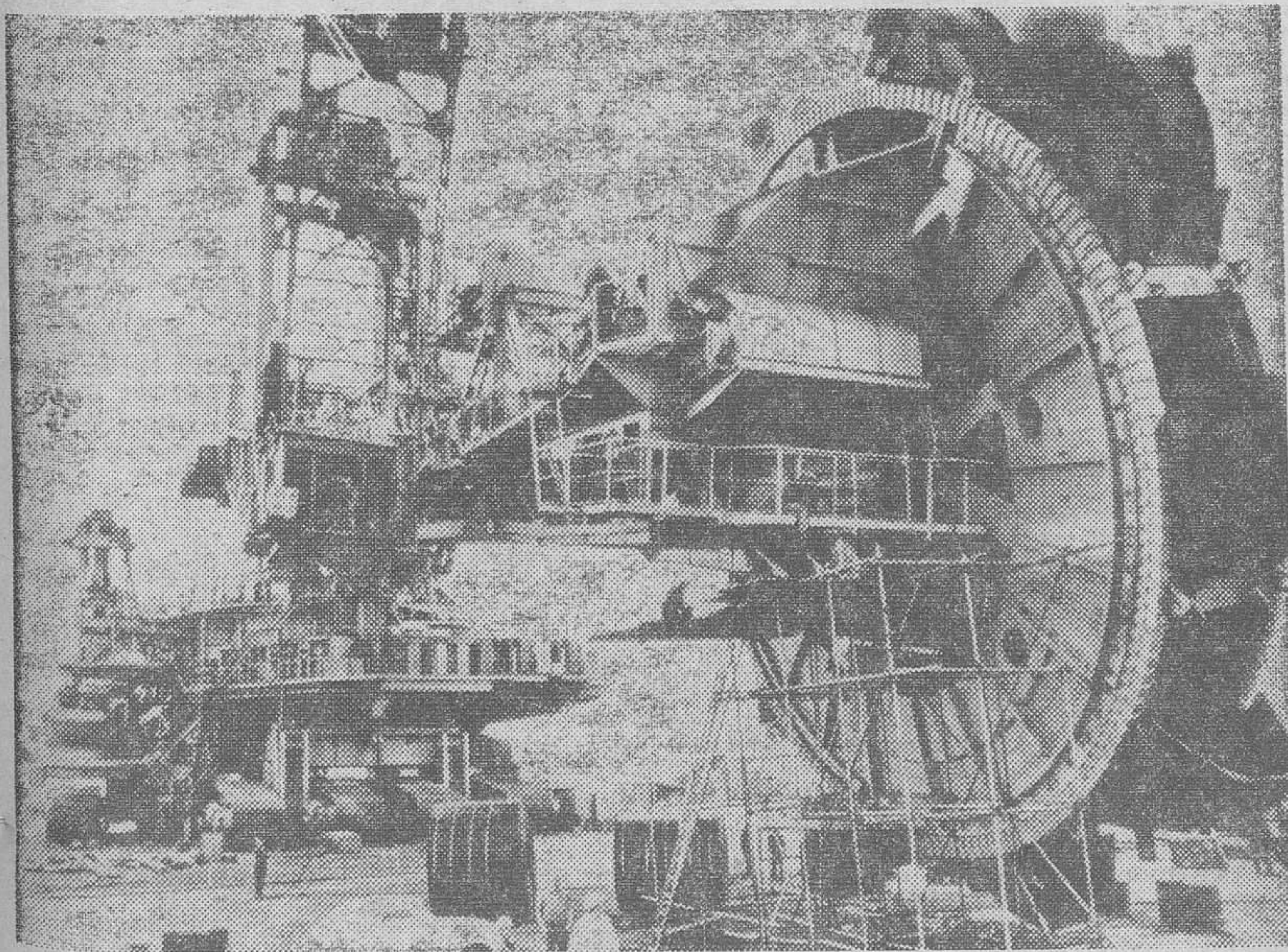
Las personas y el automóvil que vemos en la parte inferior de esta fotografía parecen figuras de juguete al lado de la gigantesca excavadora, que acaba de entrar en funcionamiento en unos yacimientos de lignito cerca de Aquisgrán, Renania (Alemania). Su rendimiento es de 110.000 metros cúbicos al día. Desde la crisis energética, la importancia del lignito, la fuente de energía primaria más barata de Alemania, ha vuelto a aumentar. En la región comprendida entre Colonia, Düsseldorf y Aquisgrán están los mayores yacimientos de lignito de Europa, calculados en unas 55.000 millones de toneladas. De las 120 millones de toneladas extraídas en 1973, el 85 % fue empleado para la obtención de corriente eléctrica. — (Foto FIEL)
