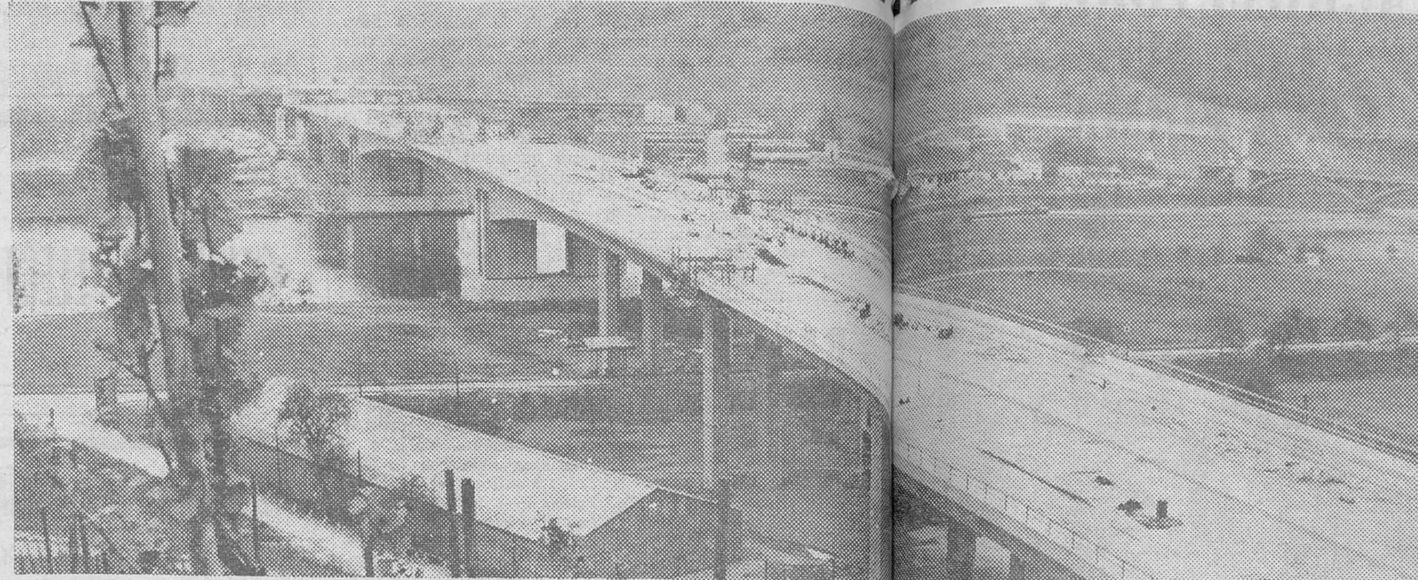
Este puente sobre el río Mosel, al Este de Tréveris, que estará terminado a fines del verano, es uno de los más largos de la Autopista de Europa, con 930 metros. Cuando entre en servicio aliviará considerablemente las precarias y hasta catastróficas condiciones de tráfico en esta zona. — (Foto FIEL).
