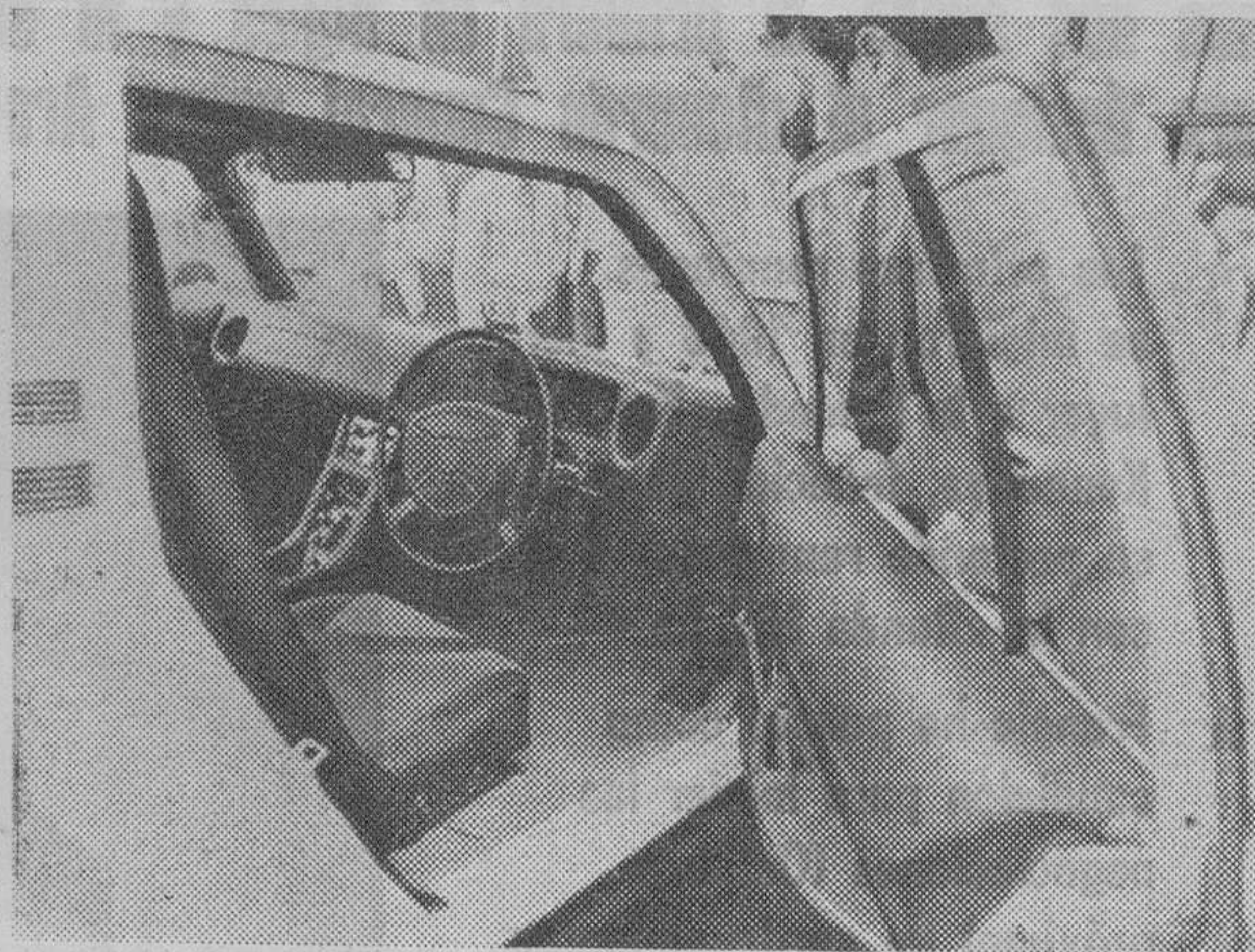
Tokio. — Los primeros vehículos experimentales de seguridad japoneses, creados conjuntamente por las fábricas "Nissan" y "Toyota", acaban de ser entregados al Ministerio de Comercio e Industria Internacional, para ser sometidos a prueba. El "Toyota" es un vehículo de dos asientos con parachoques especiales que absorben la fuerza del impacto en cualquier accidente. Dispone de bolsas de aire y un sistema especial de radar para prevención de choques. — (Foto Cifra Gráfica)
