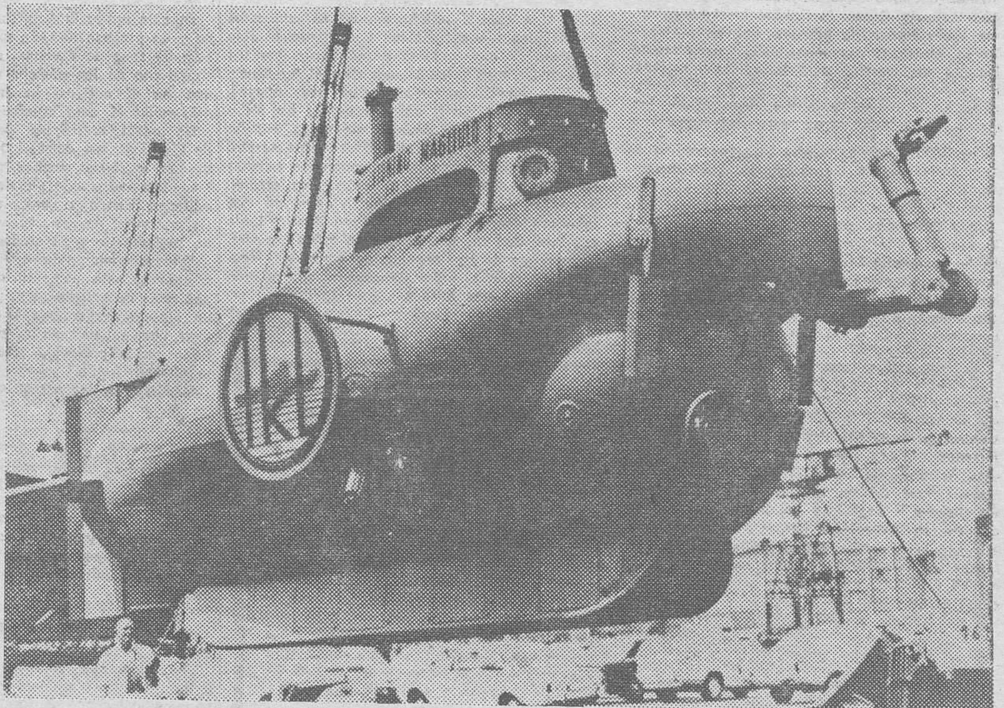
Submarino para la recogida de corales en el Mediterráneo. Ha sido diseñado en la República Federal de Alemania y tiene un radio de acción de 40 kilómetros. — (Foto LOGOS).
