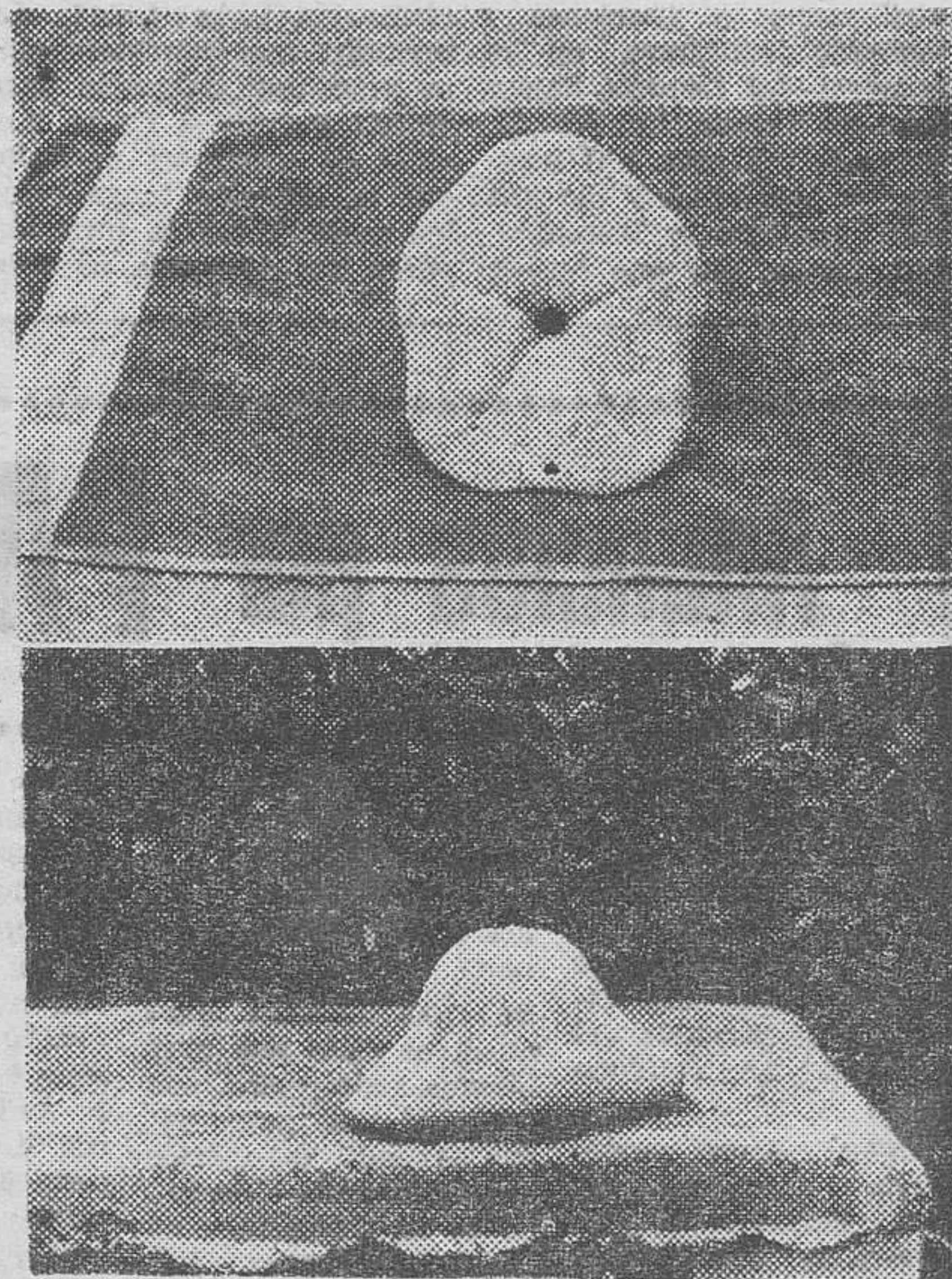
Equínida, cogido en La Serreta (Alicante) en posición normal y visto por la parte inferior, del museo de D. Isaac Rodríguez de Lera, en Aranda de Duero.
