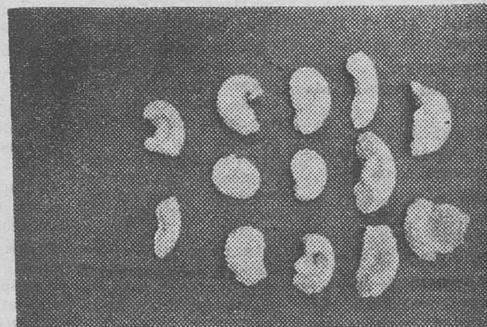
Ammonites, cogidos en La Serrezuela (Segovia)
