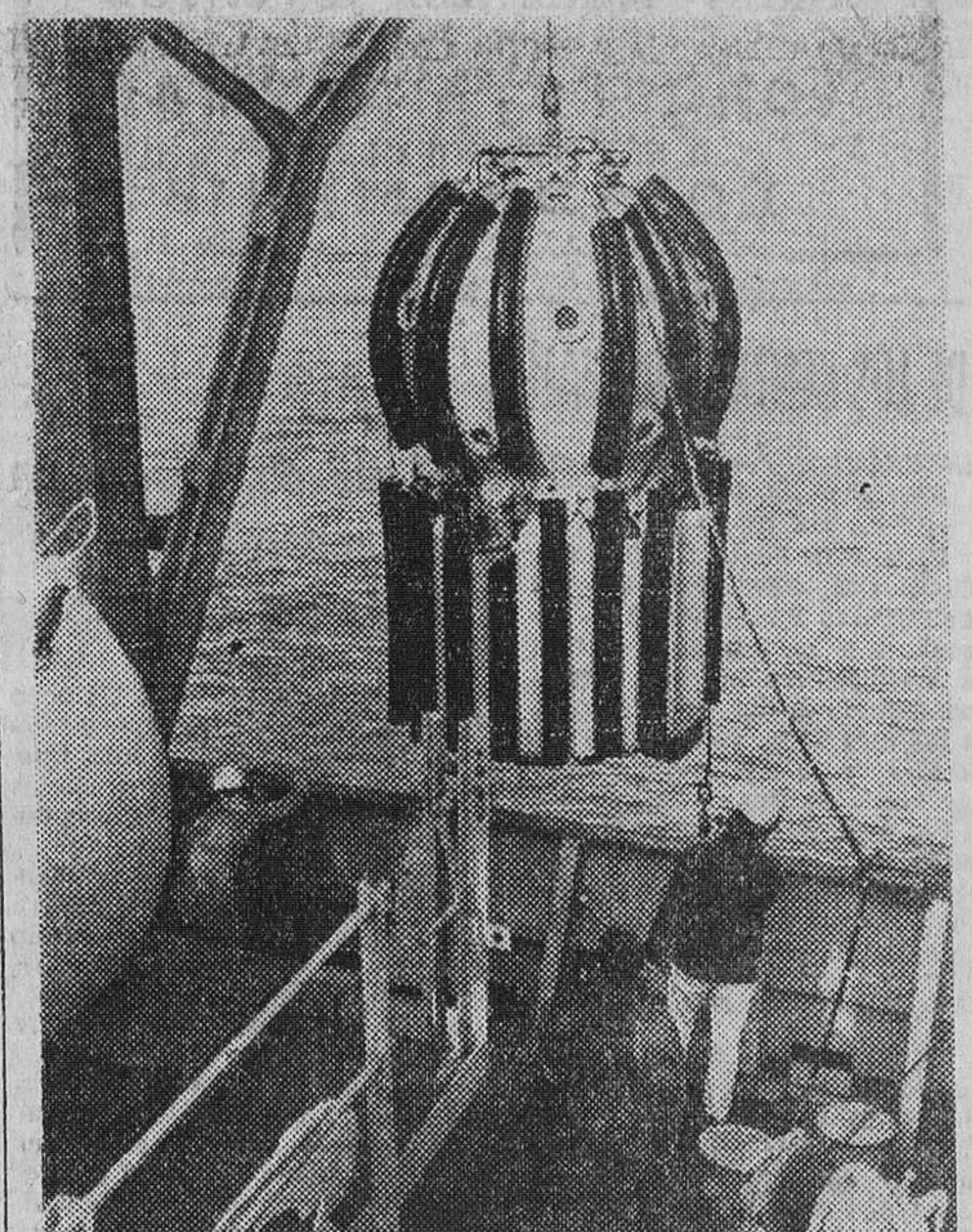
En el momento de ser introducido en el mar el buque «Orion» vemos en esta foto el batiscafo inglés «Sea Bed Vehicle» (vehículo del fondo del mar), construido por una firma británica que ha intervenido en la exposición internacional de Oceanología 1969 celebrada recientemente en Inglaterra. Barcos especiales de reconocimiento e investigación de Gran Bretaña, Rusia, Estados Unidos y Polonia presenciaron las pruebas desde lugares cercanos. — (Foto FIEL)
