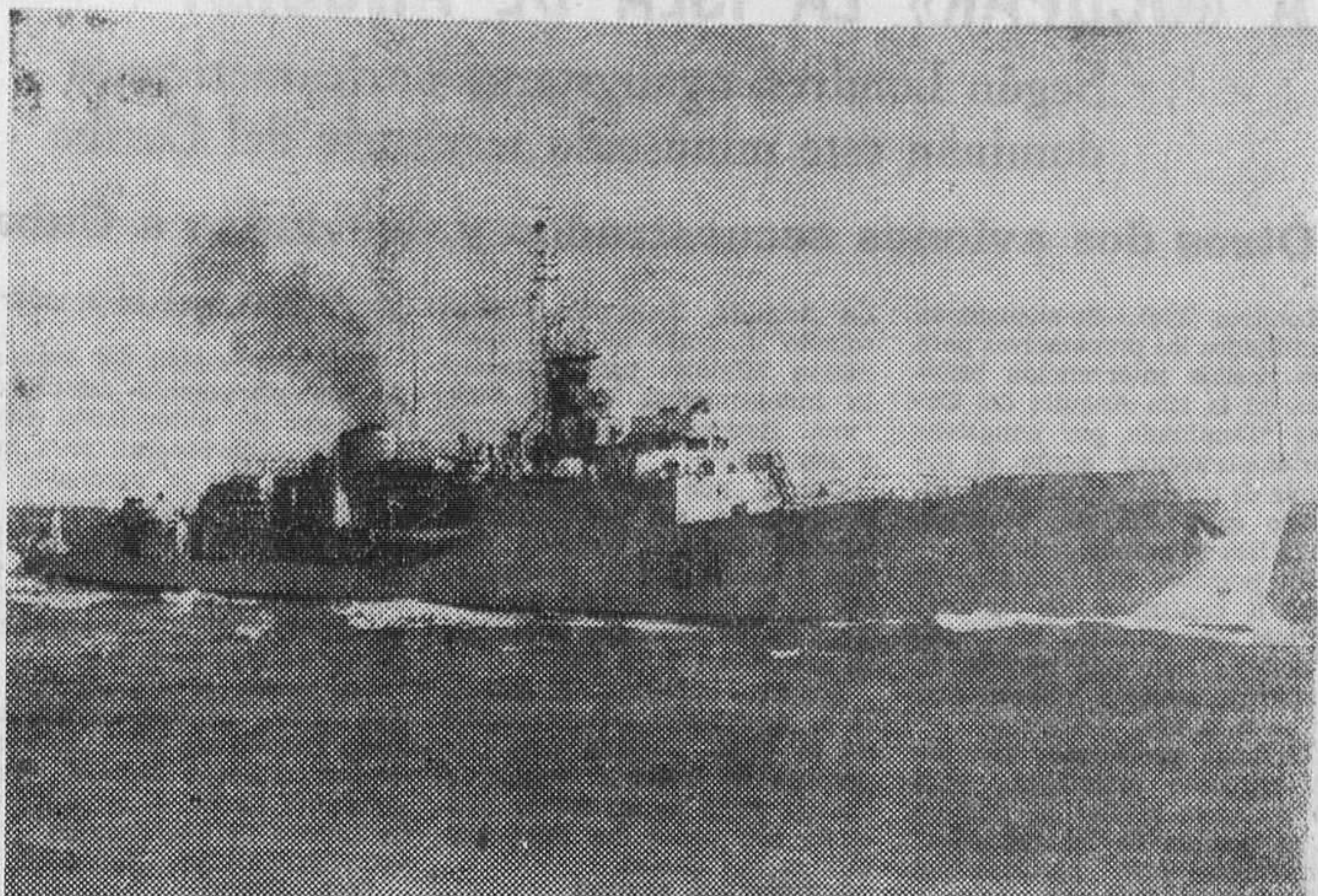
Este es el «Exmouth», el primer buque con todas sus turbinas de gas, fotografiado en el Canal de Inglaterra, fuera de Portsmouth, en el momento de iniciar un viaje hacia varios puertos escandinavos. El «Exmouth» es mandado por el comandante Brian Outhw. — (Foto FIEL)
