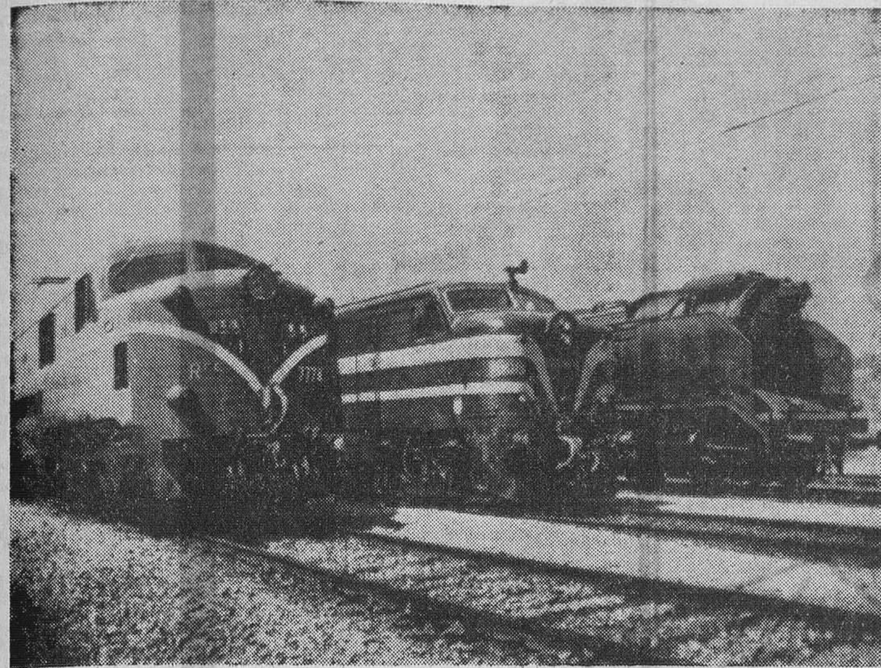
Estos son los tres sistemas de tracción empleados hoy por la RENFE. De izquierda a derecha, máquina eléctrica, máquina diesel de gas-oil o fuel-oil y máquina de vapor. — (Foto CIFRA)
