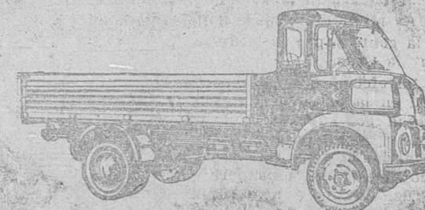
"S-66" Equipado con MOTOR DIESEL BMC (2.2) POTENCIA 56 CV. a 3.500 r.p.m. 4 VELOCIDADES adelante y marcha atrás. CAPACIDAD de carga 2 TONELADAS.
