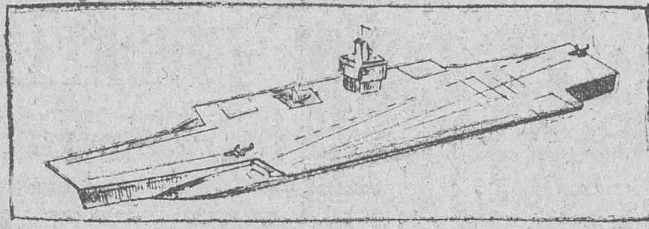
Esquema oficial del "Enterprise". He aquí el primero de los portaaviones nucleares del mundo que acaba de ser botado en Newport, Virginia, para la U. S. A. Navy. Un barco capaz de dar veinte veces la vuelta al mundo—800.000 kilómetros— sin repostar; que transportará cien aviones capaces de portar bombas atómicas o de hidrógeno; de 280.000 caballos de fuerza y que costará al Tio Sam la friolera de 26.100 millones de pesetas.
