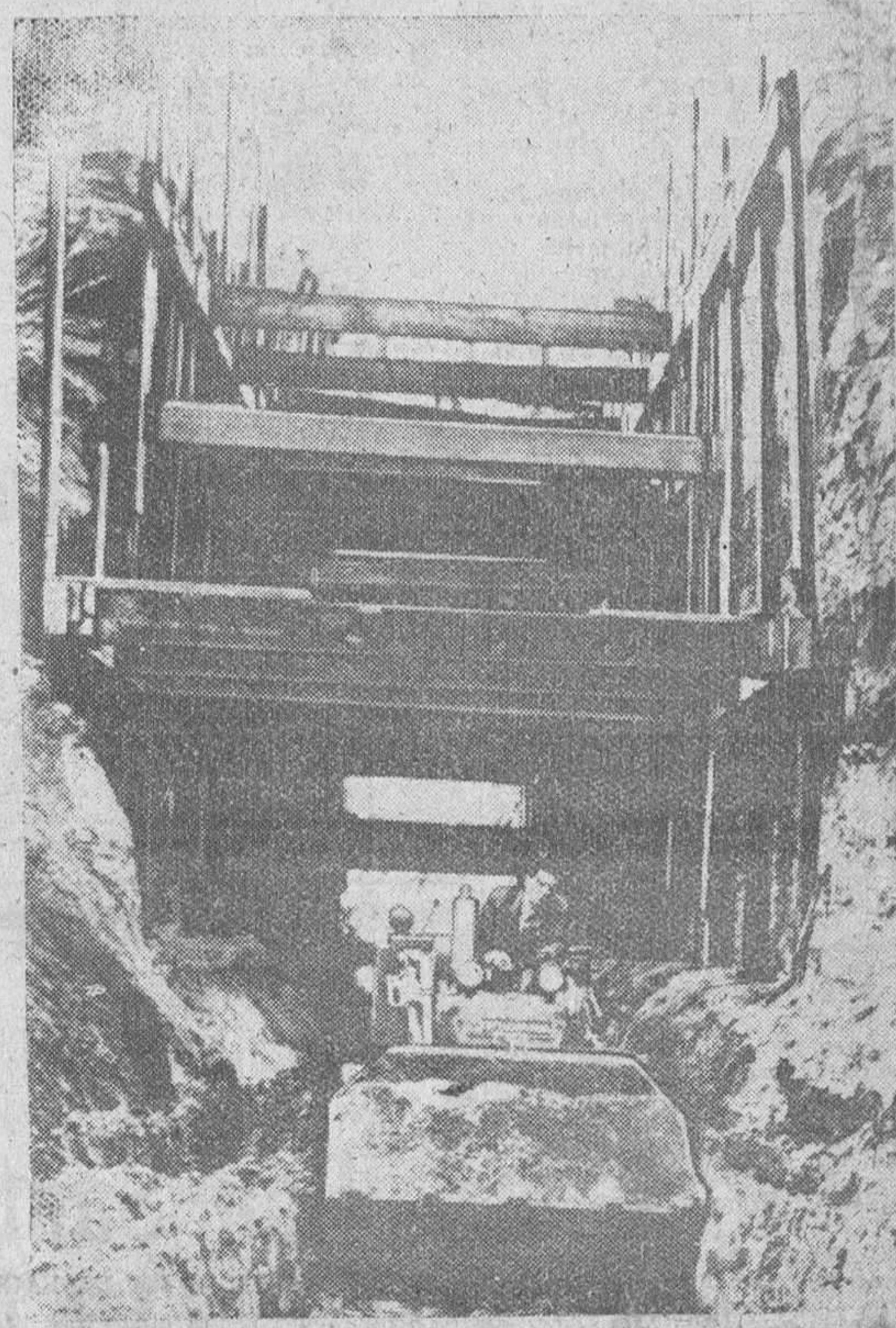
En Farnham (Inglaterra) esta máquina cortó con toda precisión un monte para permitir el paso de una nueva carretera. Comenzando desde la parte más alta, la máquina trabajó en secciones de sesenta centímetros de profundidad hasta alcanzar el nivel necesario. En pocos días de trabajo, removió y cargó en camiones, 1.500 metros cúbicos de tierra, sin equipo auxiliar alguno.—(Foto Gil del Espinar)
