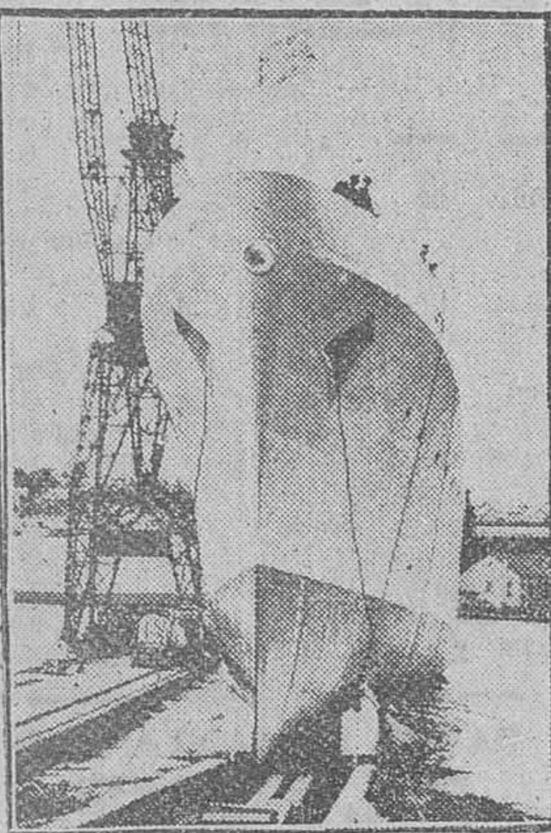
Botadura de la nueva fragata antisubmarina de la Armada británica, "Grafton" verificada en Cowes, en la isla de Wight. Mide 310 pies de eslora y 33 de manga, y armada por tres cañones "Bofors" y dos baterías de tres morteros antisubmarinos. (Foto Gil del Espinar)
