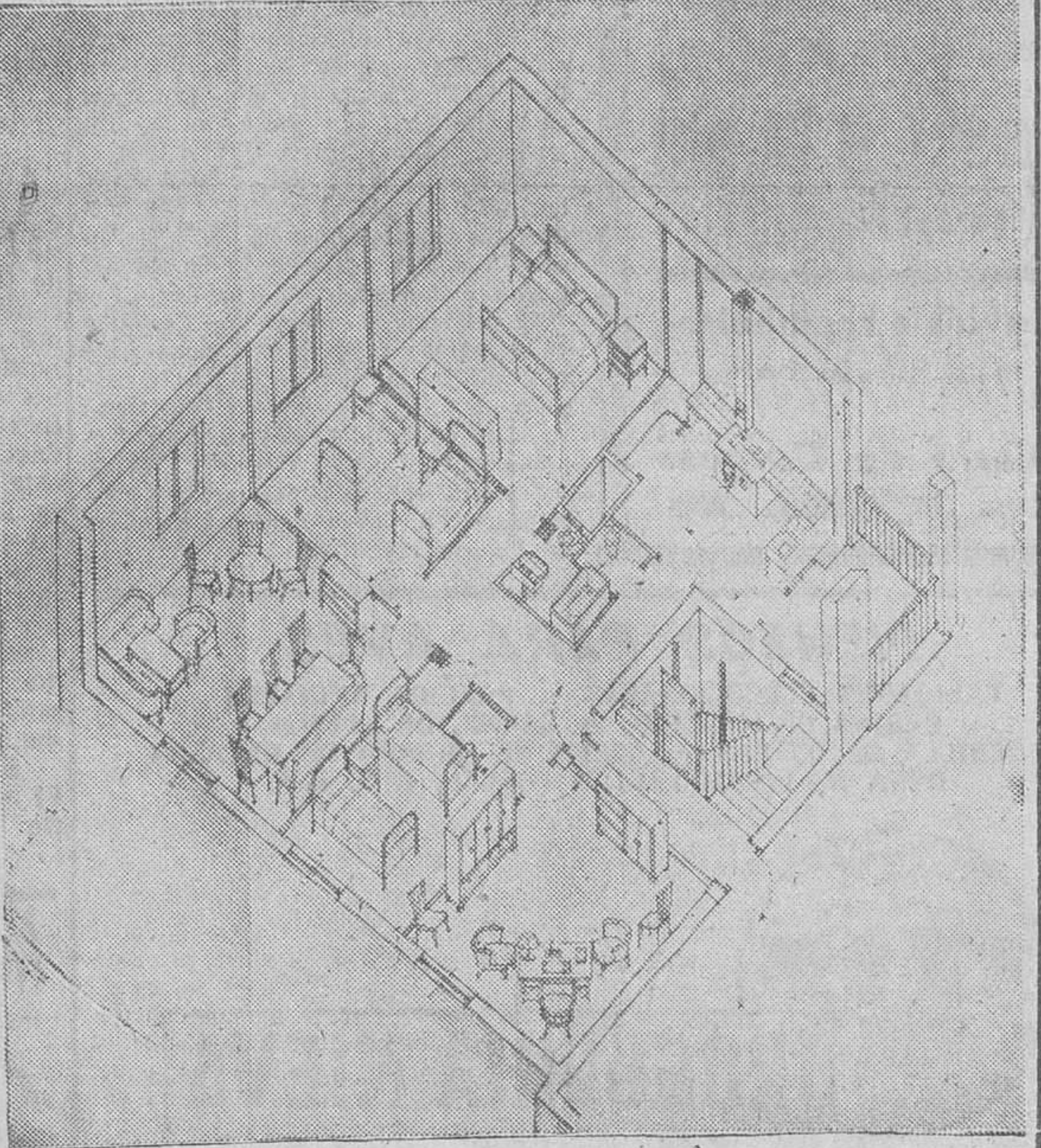
Dibujo de la disposición interior de una de las viviendas que actualmente construye la Caja de Ahorros Municipal
