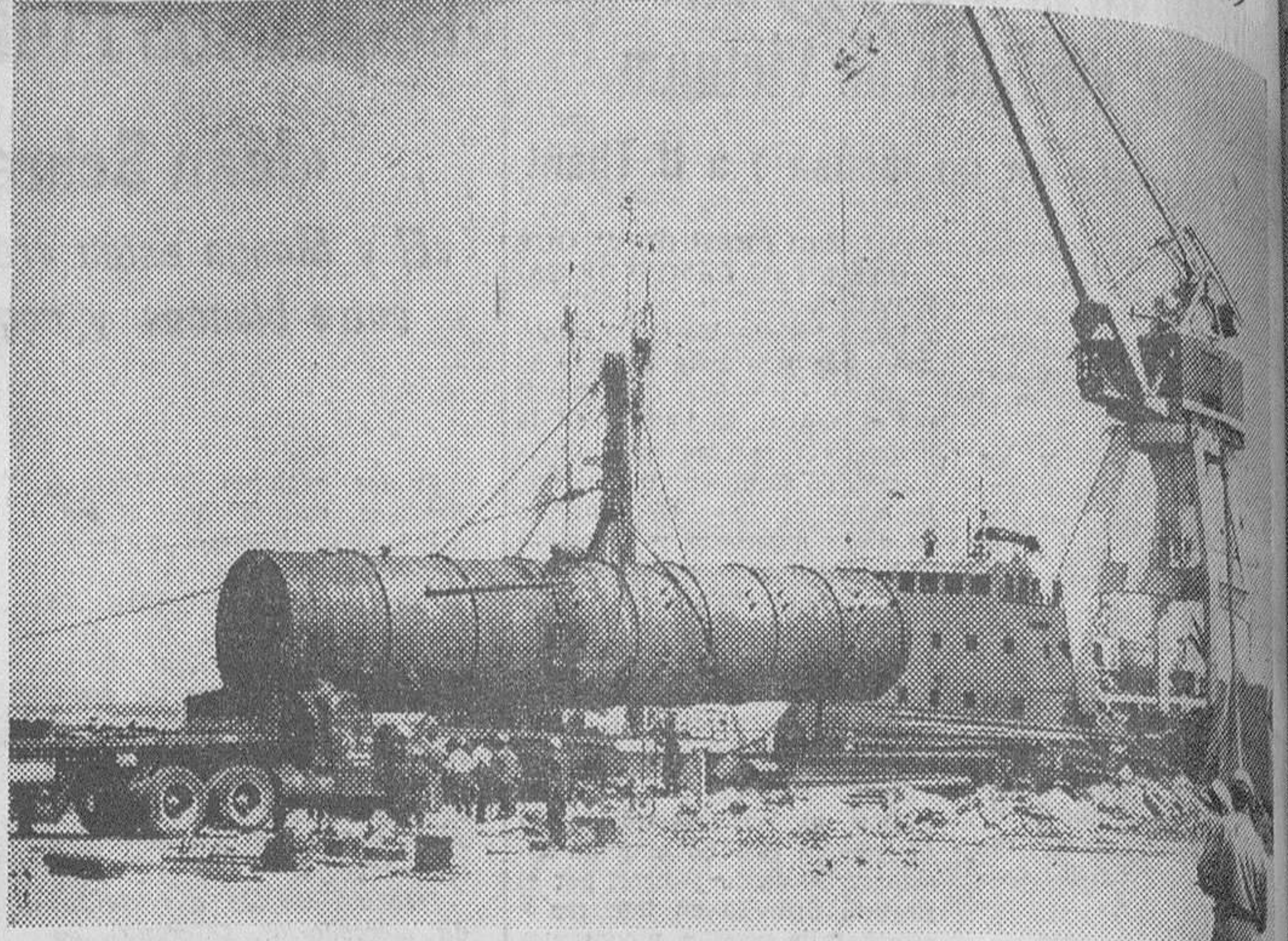
Momento de la descarga en el puerto de Algeciras de diverso material procedente de Italia para la refinaria de petróleo «Gibraltar», ya en funcionamiento en su primera fase y próxima a inauguración. — (Foto FIEL).
