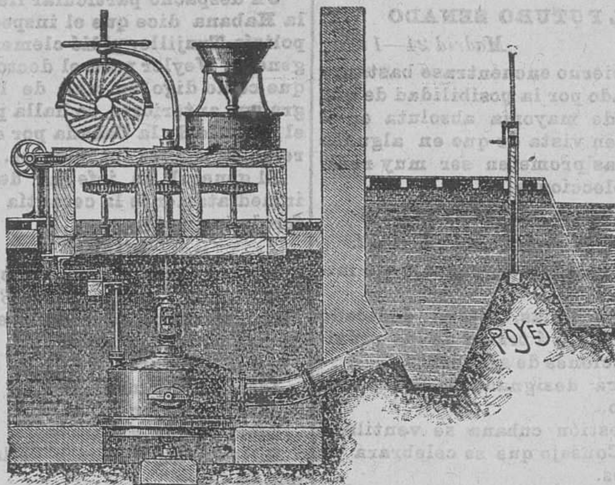
Molino de castillete de madera con turbina
