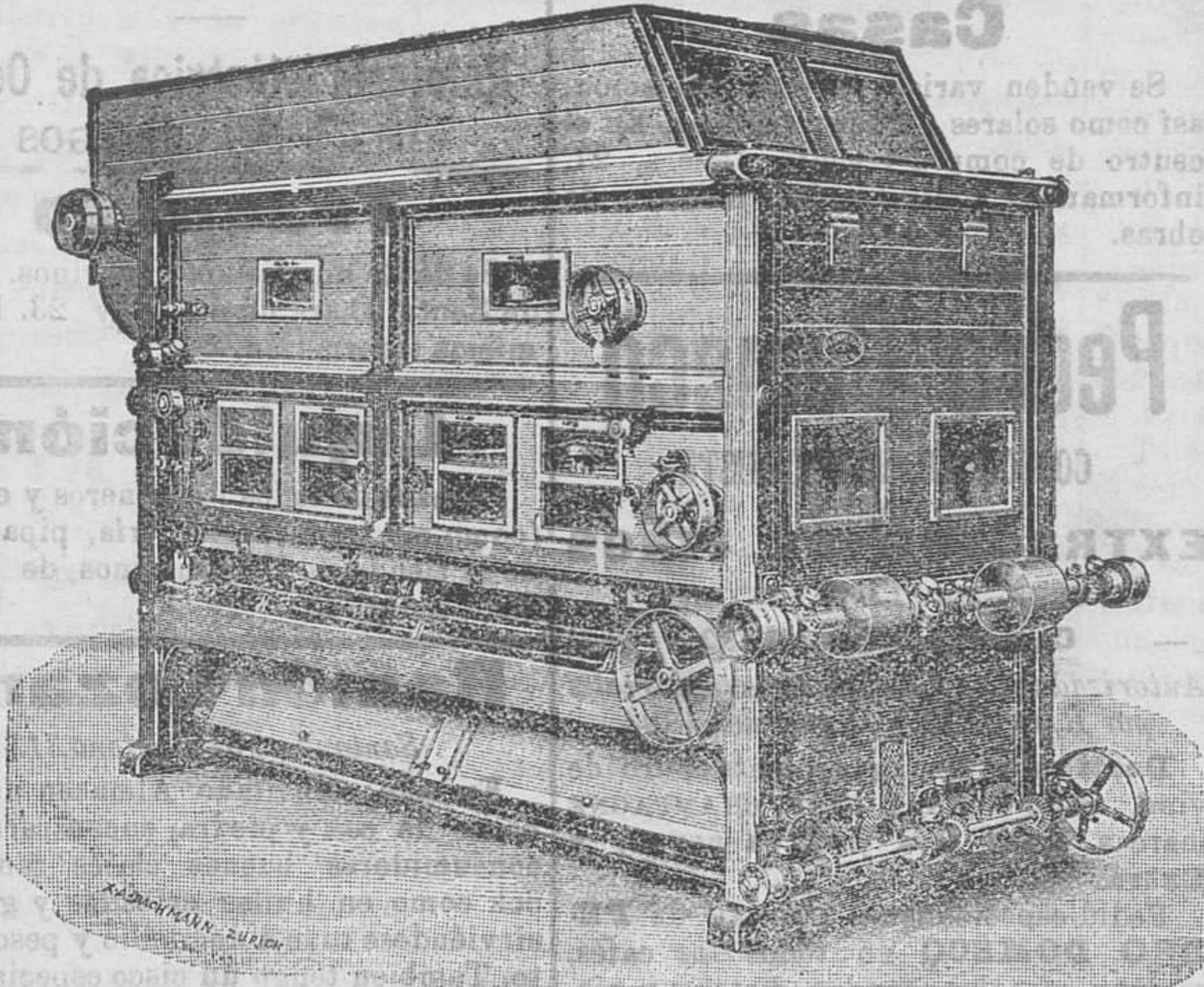
COLUMNA DESPUNTADORA
