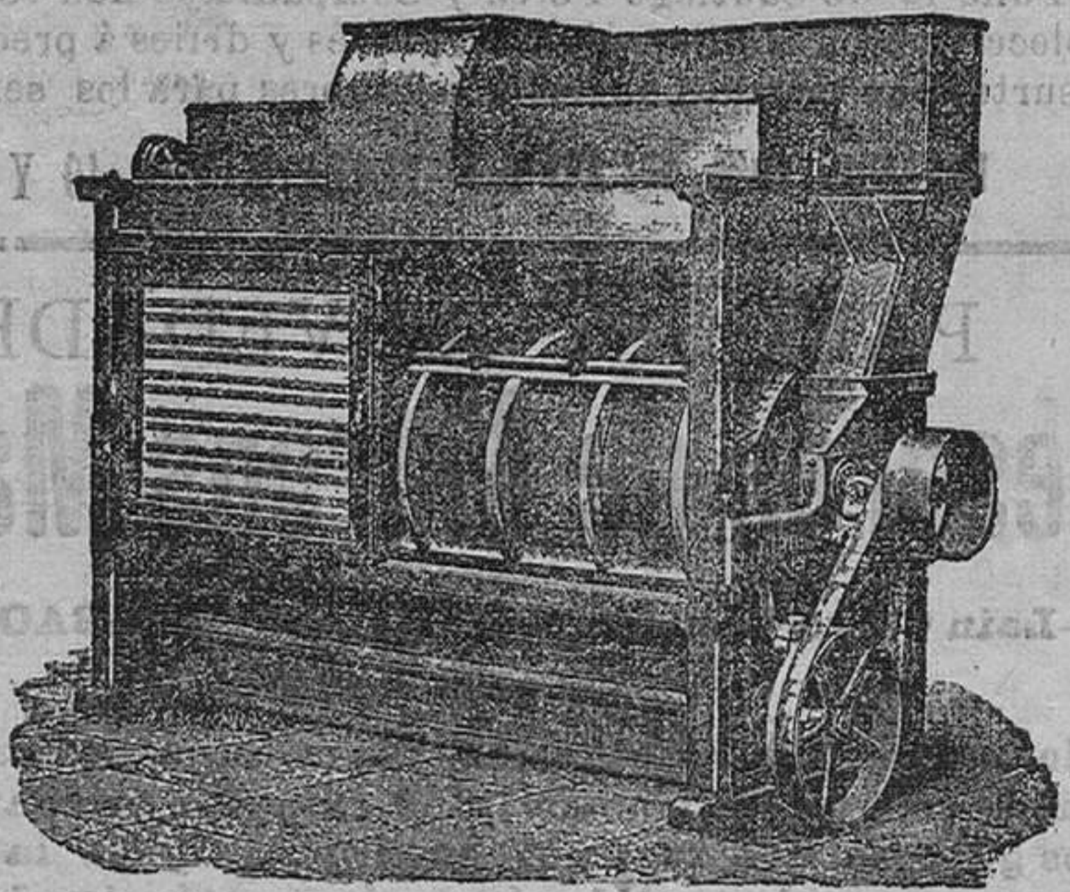
COLUMNA DESPUNTADORA
