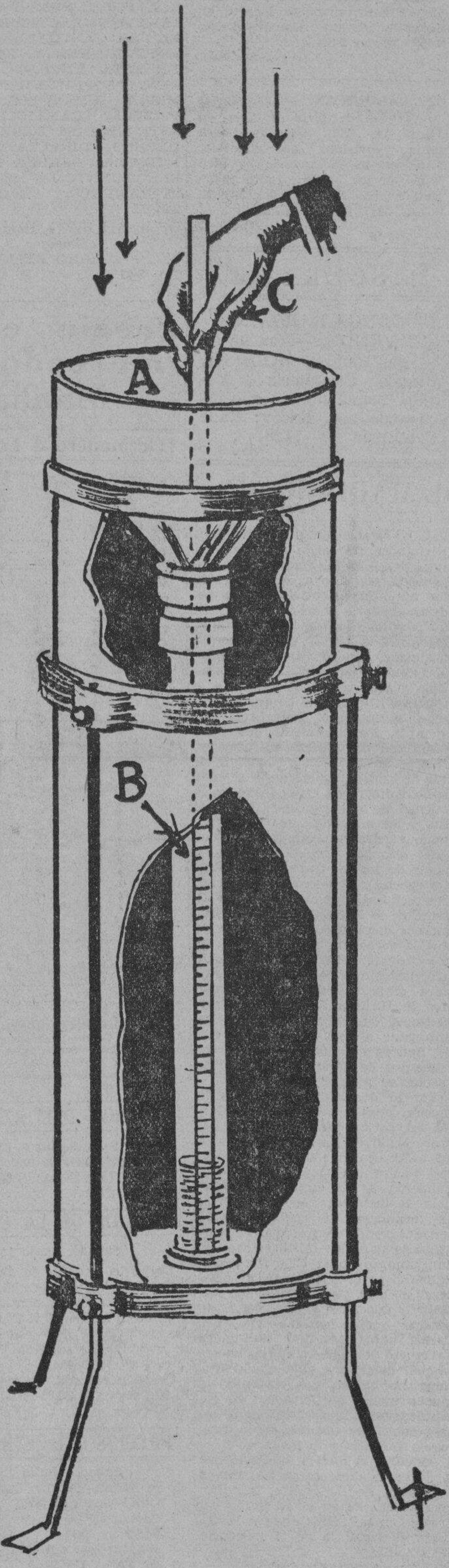
Dibujo del pluviometro de Baltimore o aparato que mide la lluvia, usado en el Observatorio de Manila. Las flechas indican las gotas de agua que caen en la vasija (indicada con la letra A) que tiene 8 pulgadas de diametro; el agua continua cayendo hasta el tubo (letra B) que mide 2.53 pulgadas. La letra "C" representa la mano del observador que coge la medida con la que se mide la cantidad de la lluvia en el tubo.
