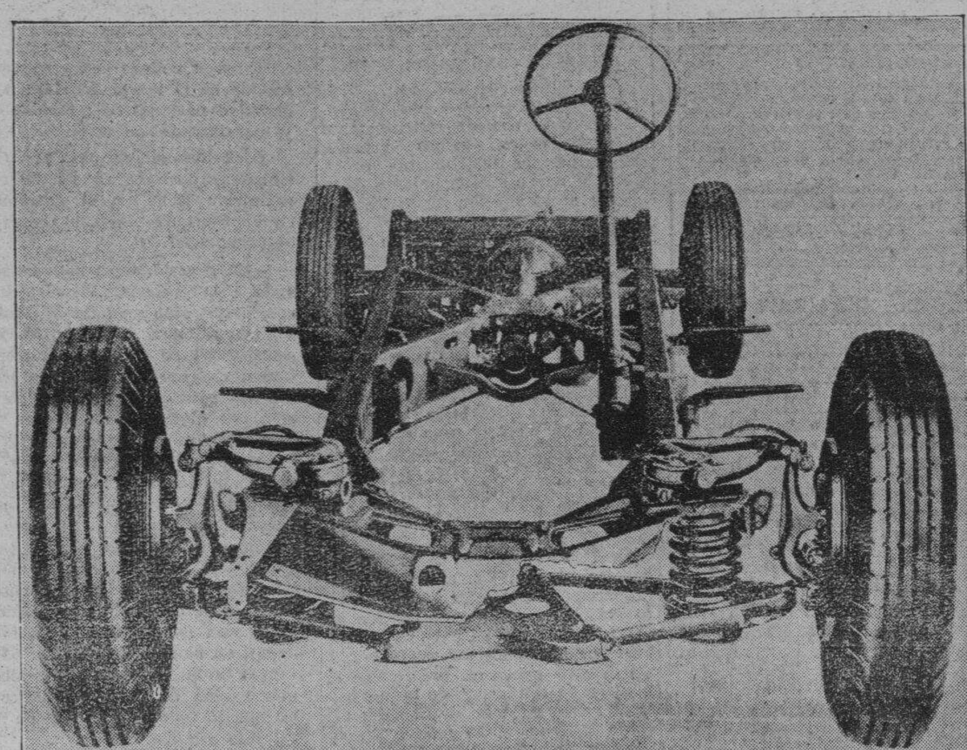
Teniendo por fase saliente una sensacional mejora en las ruedas delanteras, la llamada "knee-action", que impide que el coche de tumbos cuando la rueda tropieza con obstaculos, no elevandose levemente mas que una de las ruedas, pues el eje no es entero y soñado sino que tiene en medio un aparato que hace de una rueda independiente de la otra, la primera remesa de los Buicks de 1934 para Filipinas llegara aqui la semana proxima. Los manilenses obtendran su primera oportunidad de verlos hacia el 21 del actual, segun anuncio ayer Mr. G. M. John, gerente de la "Automotive Sales Co." La fotografia de arriba demuestra al nuevo Buick con rueda delantera con suspension independiente, que da mas comodidad a los pasajeros como nunca jamas.
