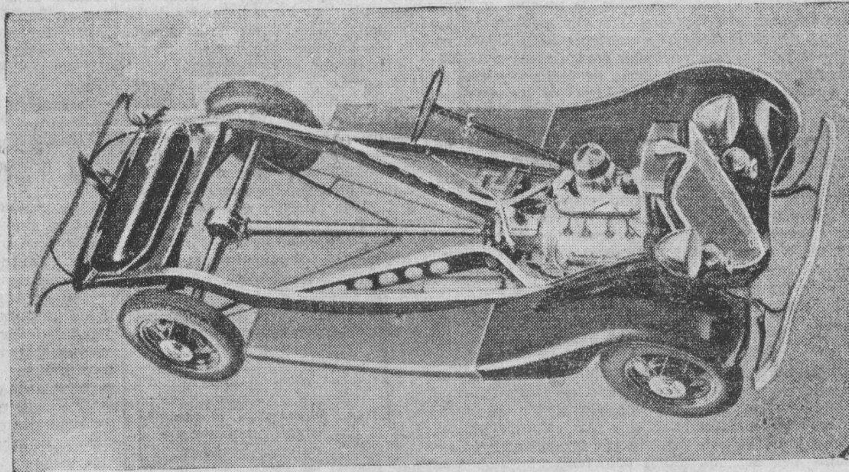
UNA VISTA DEL FONDO DEL NUEVO CHASIS FORD V-8
